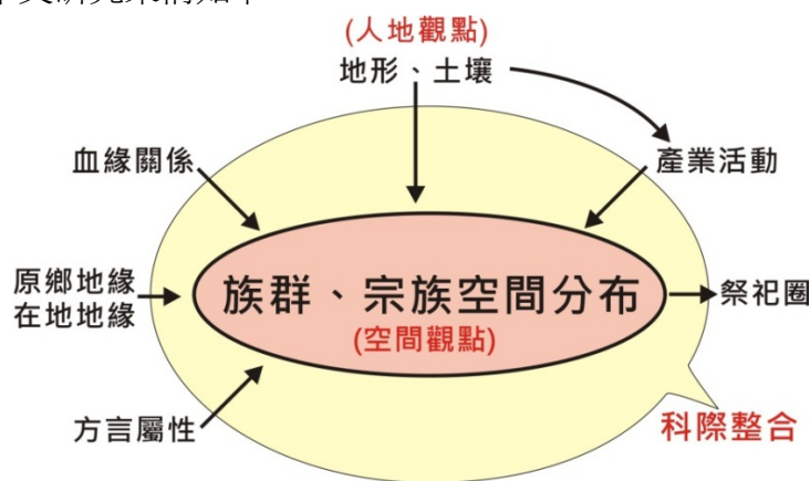
圖 1、研究架構圖
