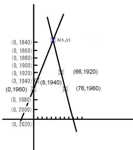
圖 4-3-1、回溯語言產生年代和地點模型
