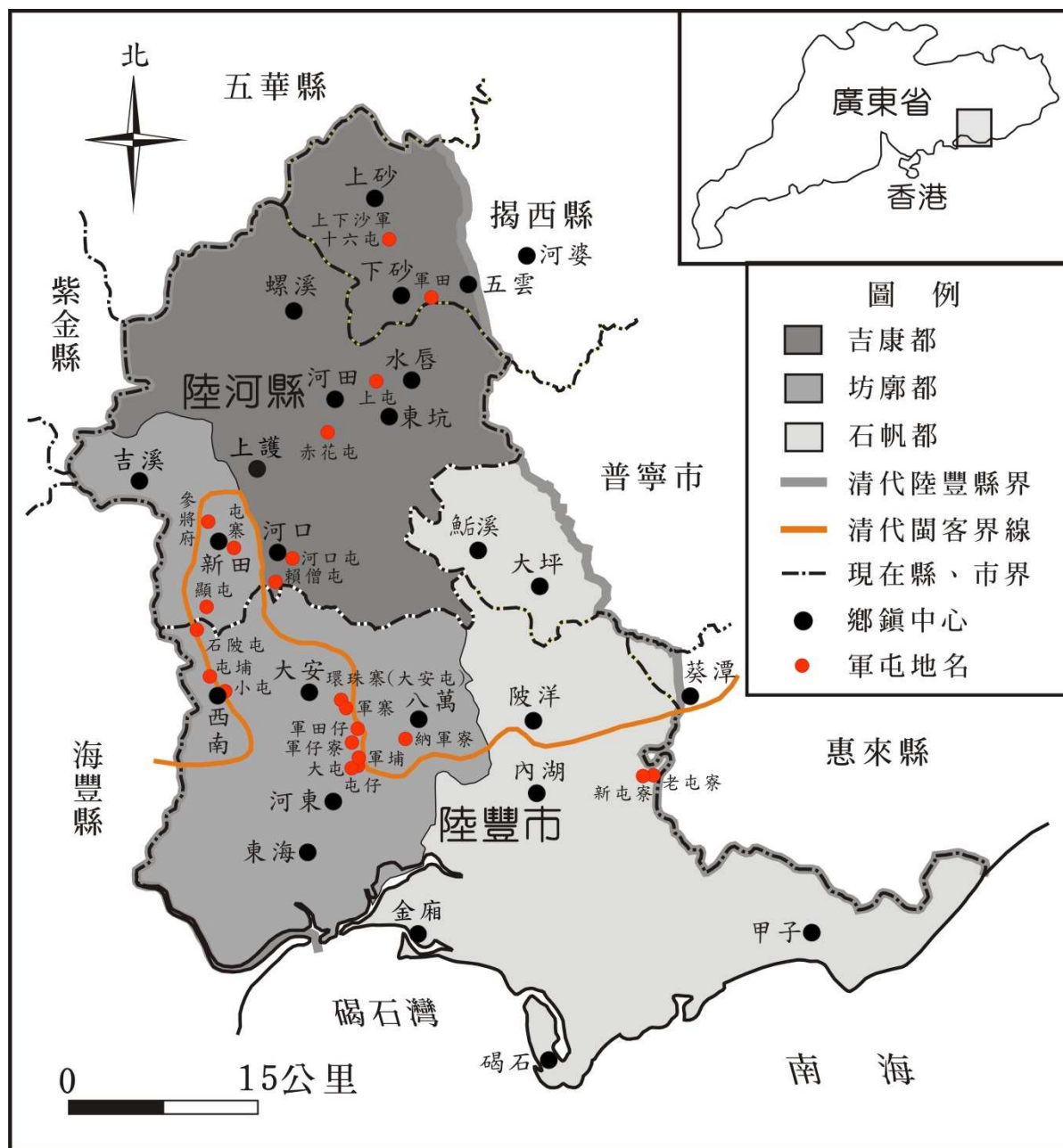
圖 6、舊陸豐縣（1731-1965 年）的軍屯地名
