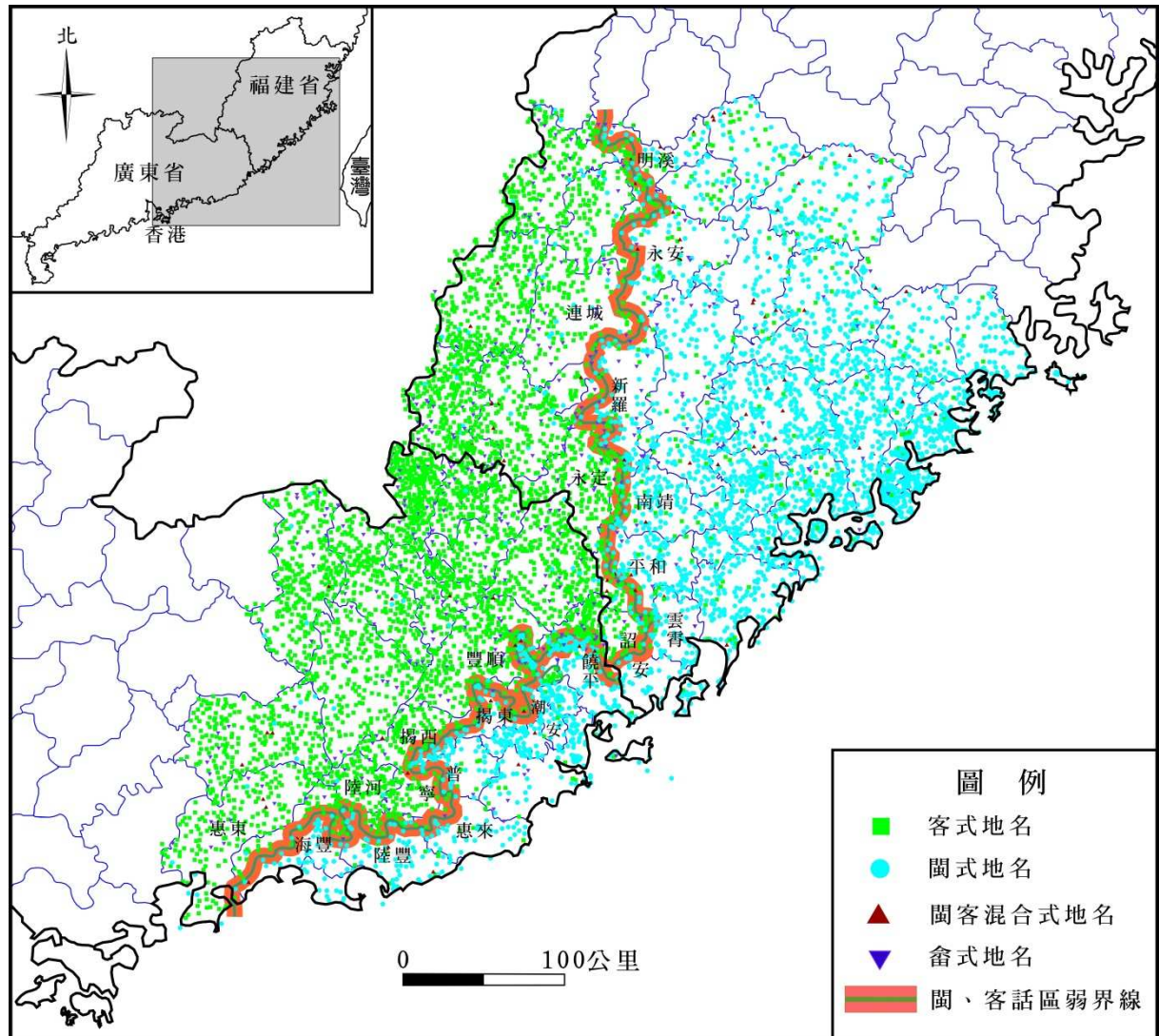
圖 2：以閩、客式地名所繪製的「閩西南及粵東閩、客歷史方言分區圖」
