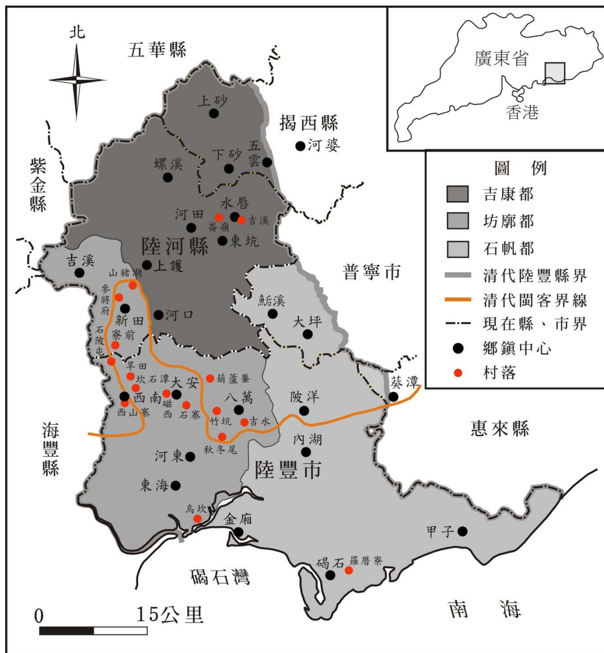
圖 5、清代陸豐縣之三都
