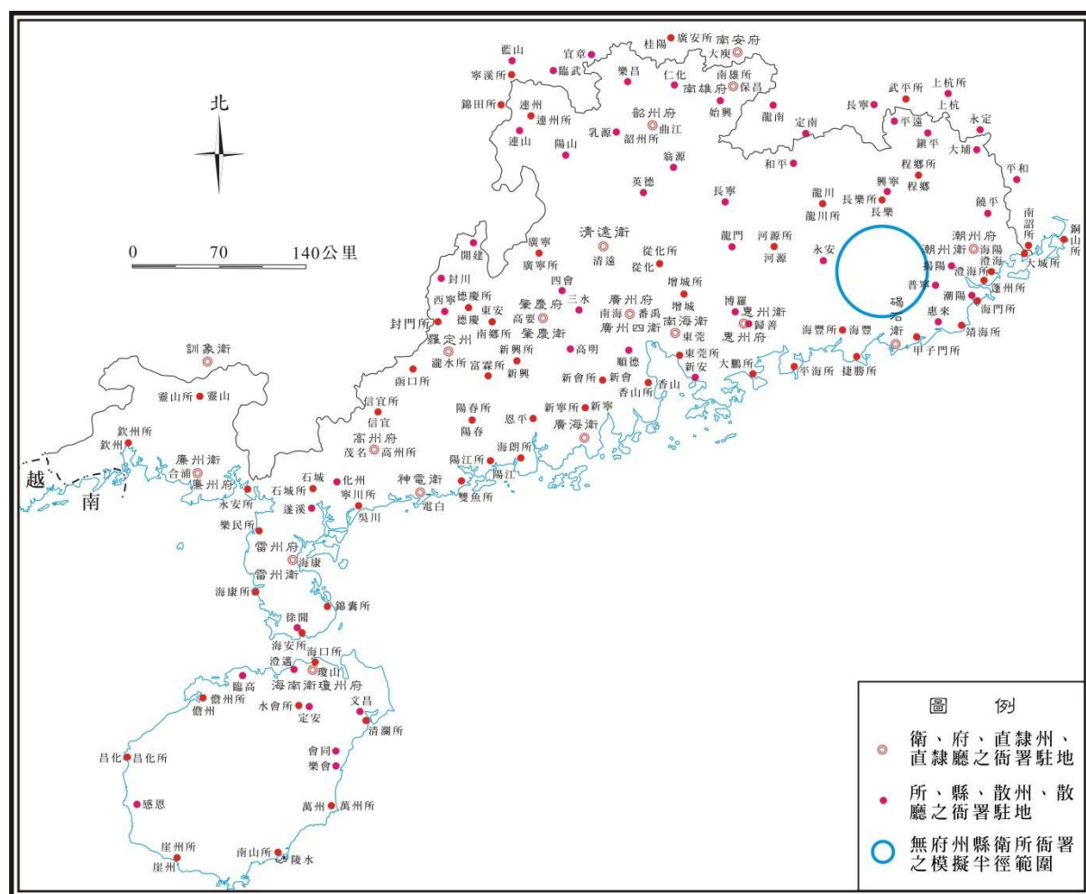
圖 4、明代廣東省衛所衛、所及府、州、縣治分布圖
