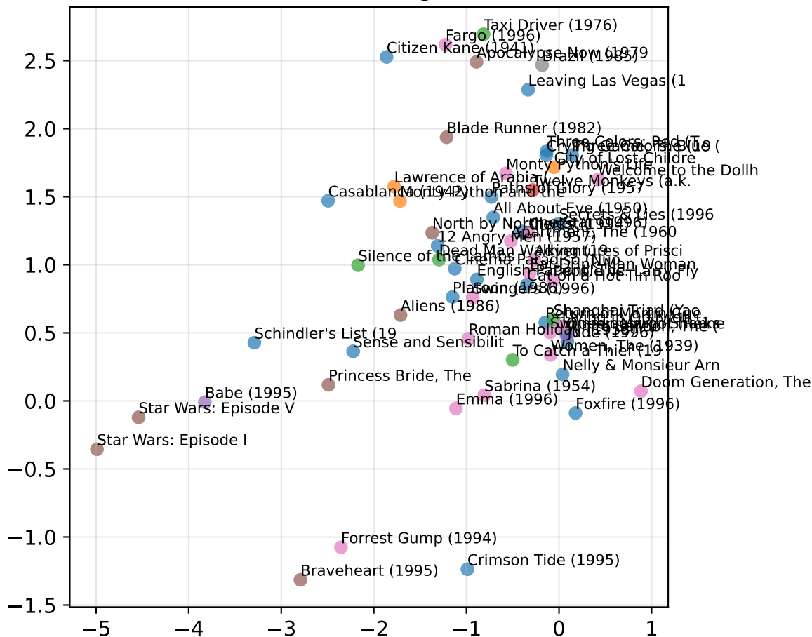
Movie Embeddings (k=2)
