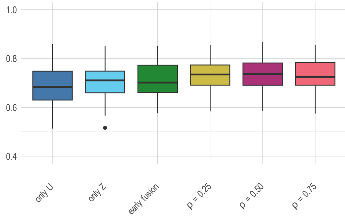
Uno C-index
