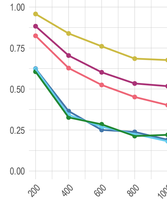
NSR
