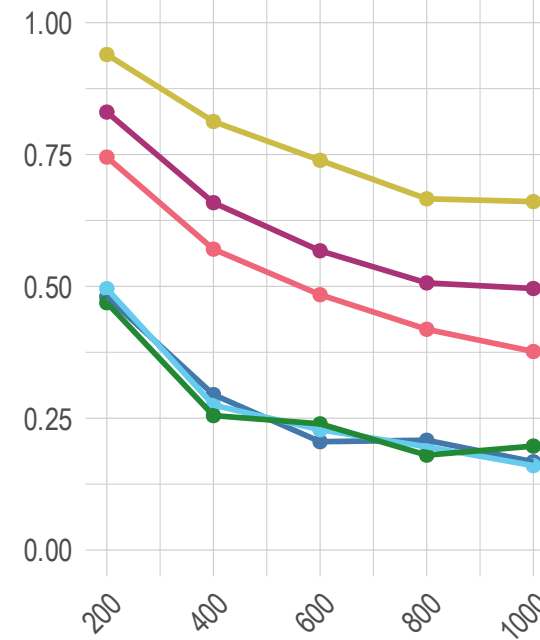
FPR
