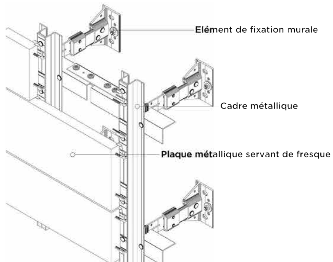
Détails fixation plaque métallique au mur
