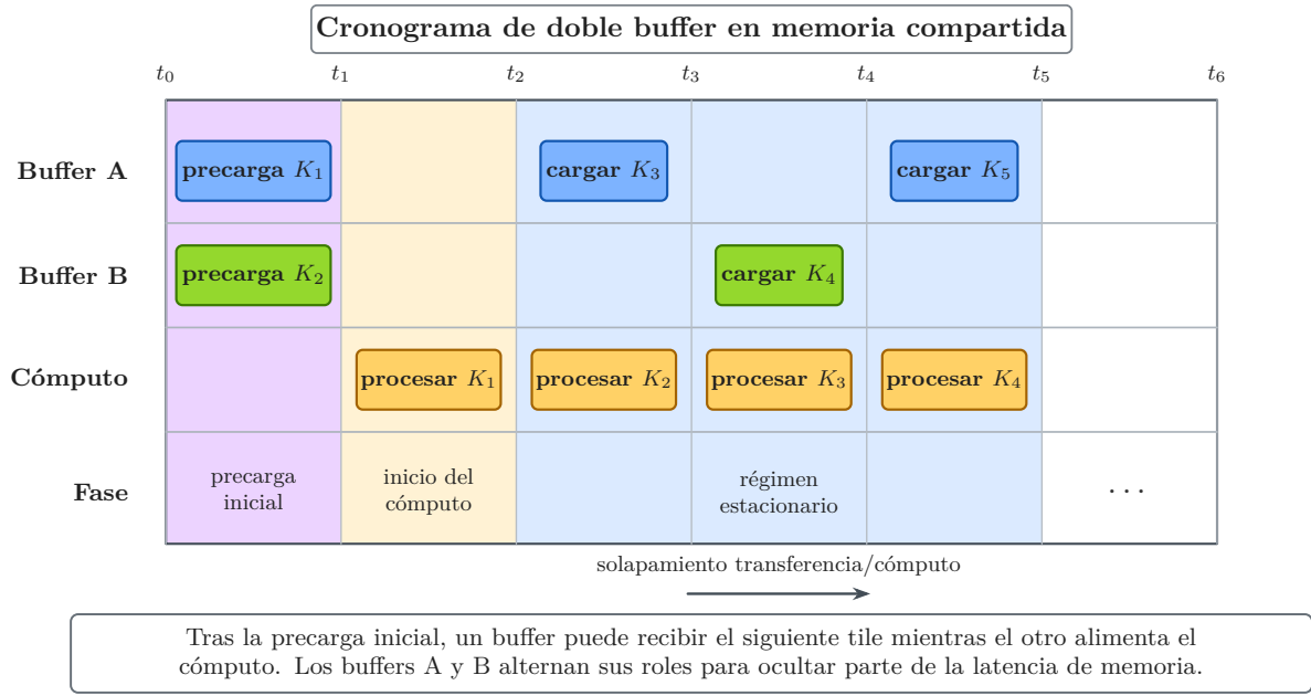
Figura 3.7. Cronograma de un multibuffer de dos etapas en SRAM. Tras la precarga inicial, una etapa puede reutilizarse para cargar los siguientes tiles K_i y V_i mientras se procesan los datos almacenados en la otra. En la imagen, solo aparecen las precargas de K para simplificar, pero en la práctica, un buffer lo forma un par (K_i, V_i)
