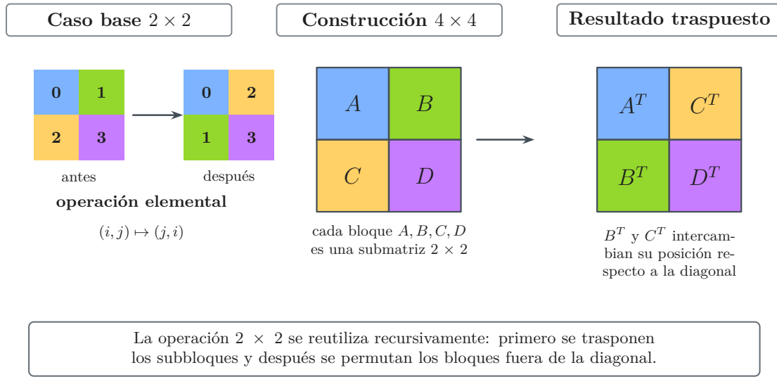
Figura 3.4. Traspuesta en registros: idea recursiva.
