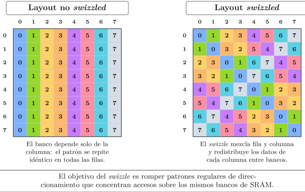
Figura 3.6. Comparación entre un layout naive y un layout swizzled en SRAM. El swizzle modifica la distribución de los elementos entre bancos para evitar conflictos de banco en el patrón de acceso considerado.
