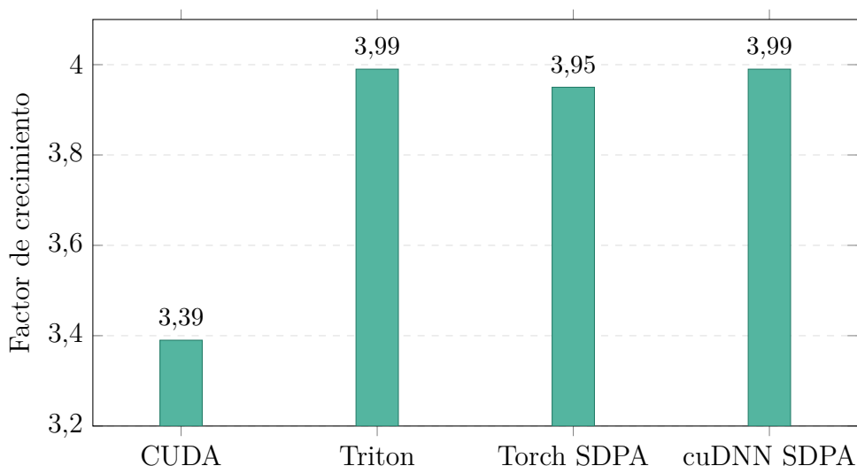
Figura 4.2. Factor de crecimiento del número de ciclos al aumentar la longitud de secuencia de 16384 a 32768.
