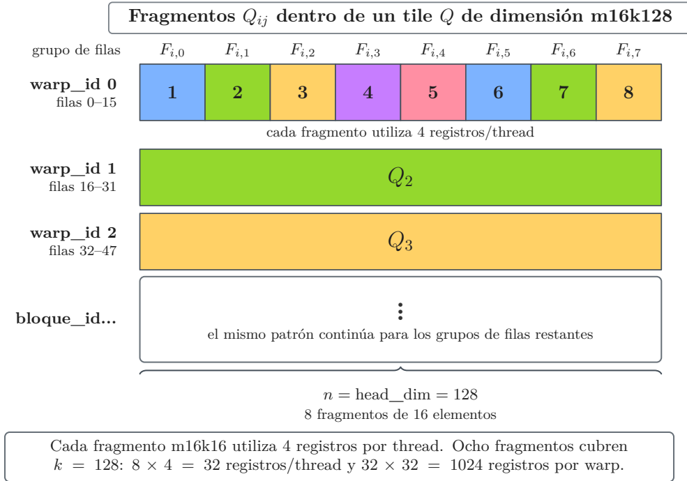
Figura 3.3. Mapping de registros para elementos de Q (m16k128) usando layout A mma.sync .
