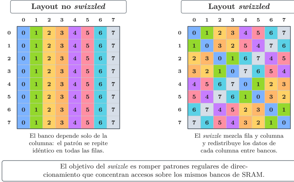
Figura 3.6. Comparación entre un layout naive y un layout swizzled en SRAM. El swizzle modifica la distribución de los elementos entre bancos para evitar conflictos de banco en el patrón de acceso considerado.
