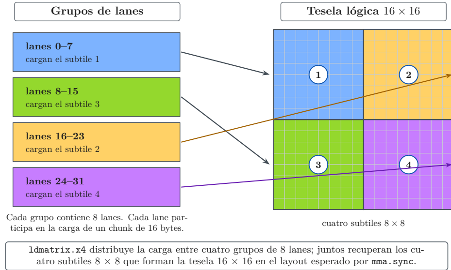
Figura 3.5. Mapeado de lanes y fragmentos en la instrucción ldmatrix.x4 para la carga de un tile 16 \times 16 desde SRAM a registros con el layout requerido por mma.sync .
