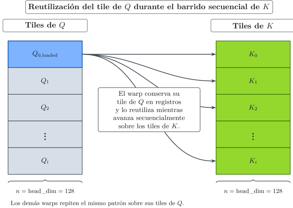
Figura 3.2. Mapping de warps: cada warp carga un tile Q y opera sobre varios tiles K_i .
