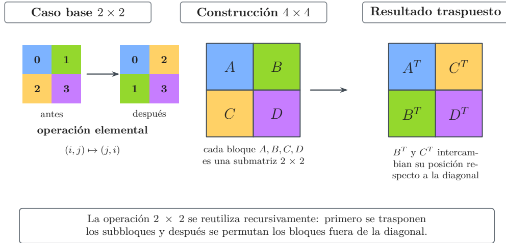
Figura 3.4. Traspuesta en registros: idea recursiva.
