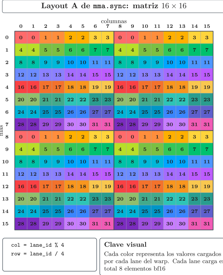
Figura 3.1. Layout A (M16×K16) para la instrucción mma.sync .
