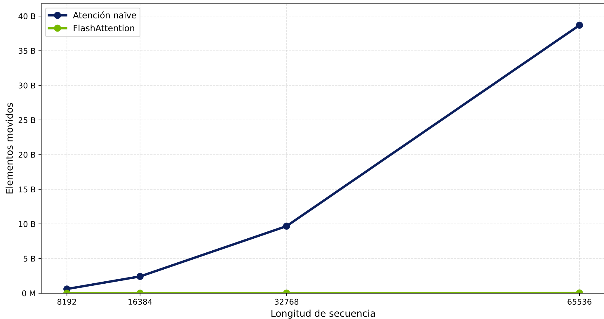
Comparativa del coste idealizado de movimiento de datos Atención naïve vs FlashAttention (head_dim = 128)
