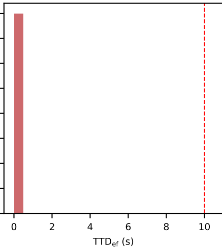
AF-TKD+MHEG
