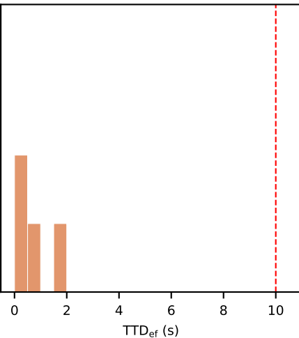
Baseline+MHEG
