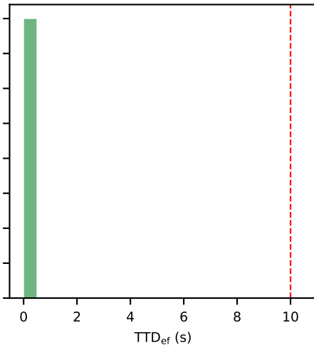
AF-TKD Fixo
