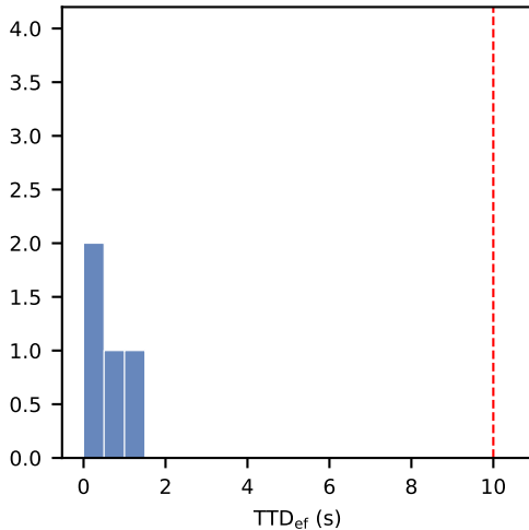
Baseline Fixo
