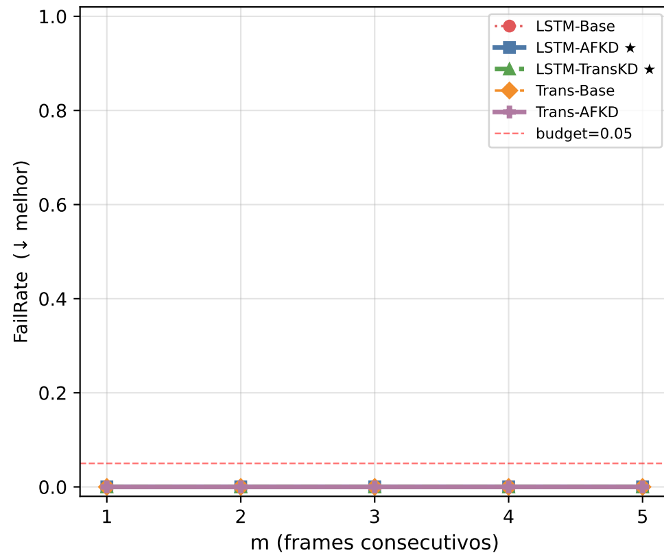
Análise 4 — Sensibilidade ao Parâmetro m (seed 45) \theta fixo = 0.100 | m \in [1, 2, 3, 4, 5] | ★ ablação: LSTM-AFKD vs LSTM-TransKD
