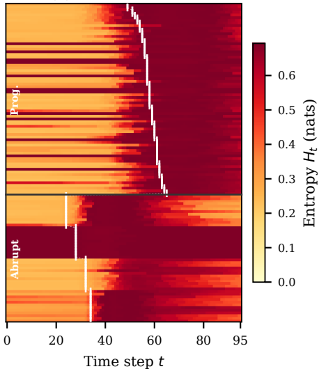
(b) AF-TOI+MHEG
