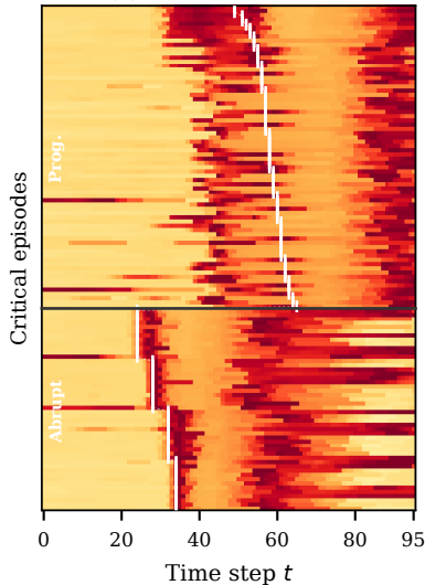
(a) Baseline+MHEG
