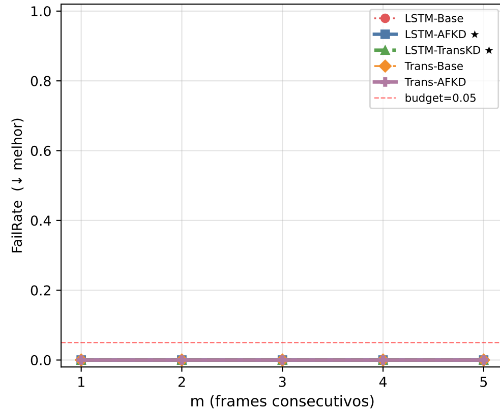
Análise 4 — Sensibilidade ao Parâmetro m (seed 43) \theta fixo = 0.100 | m \in [1, 2, 3, 4, 5] | ★ ablação: LSTM-AFKD vs LSTM-TransKD
