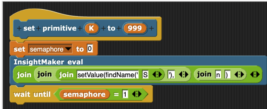
Figura 3: Bloc set primitive
