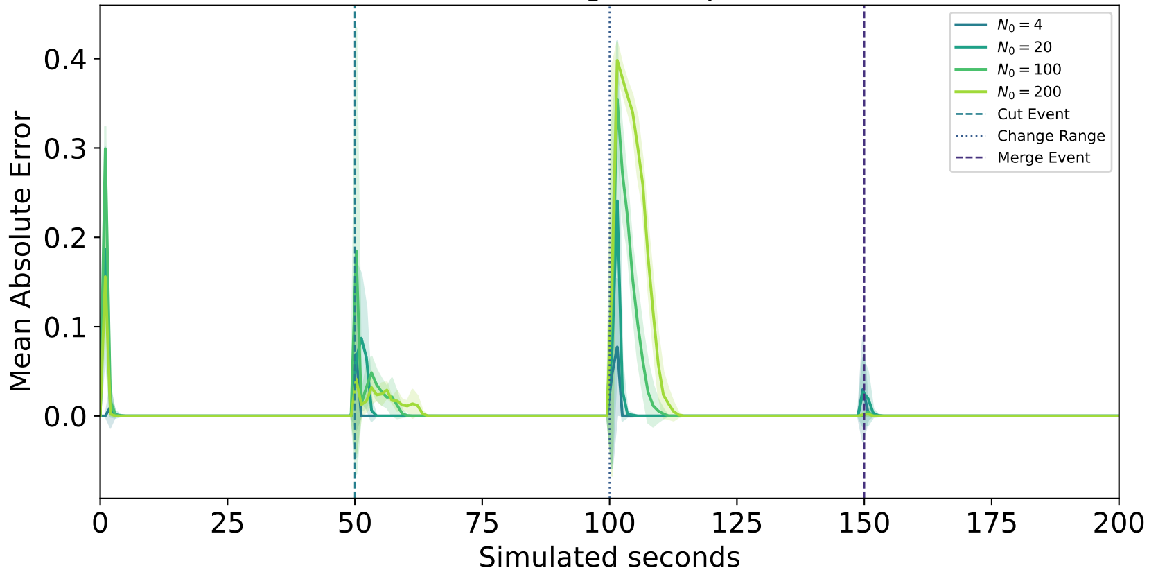
Self Stabilizing Gossip (MinOf)
