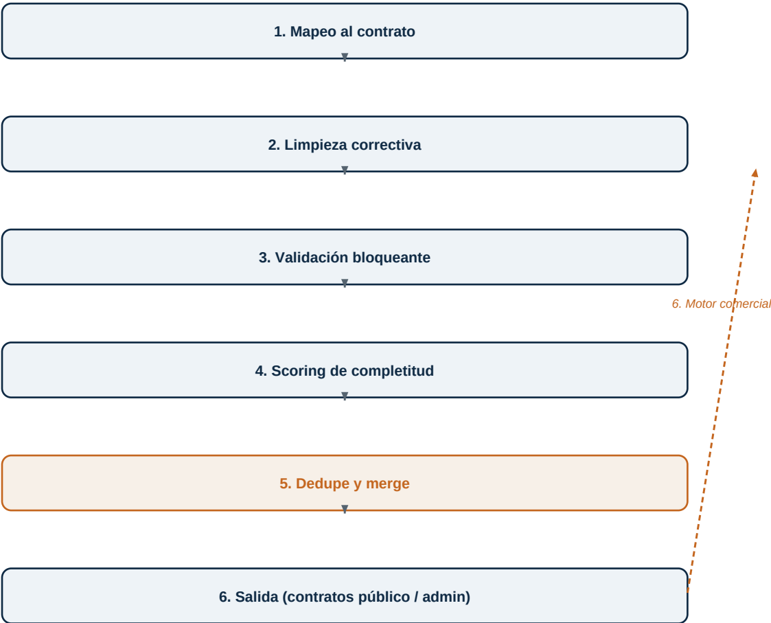
Figura 3 — El normalizador como pipeline: cada etapa acumula marcas de calidad sin detenerse, salvo en reglas bloqueantes. El motor comercial (margen + envío) corre después, sobre lo que sí se publica.
