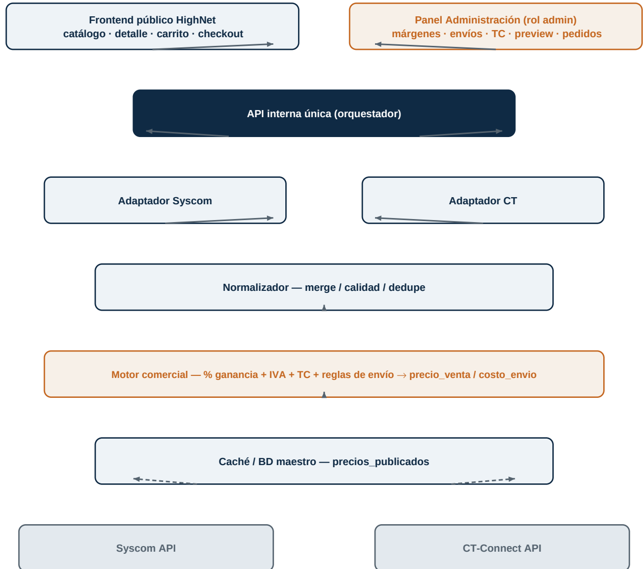
Figura 1 — Actores. El frontend público y el panel admin consumen la misma API con contratos distintos; el motor comercial ahora resuelve margen y envío juntos.
