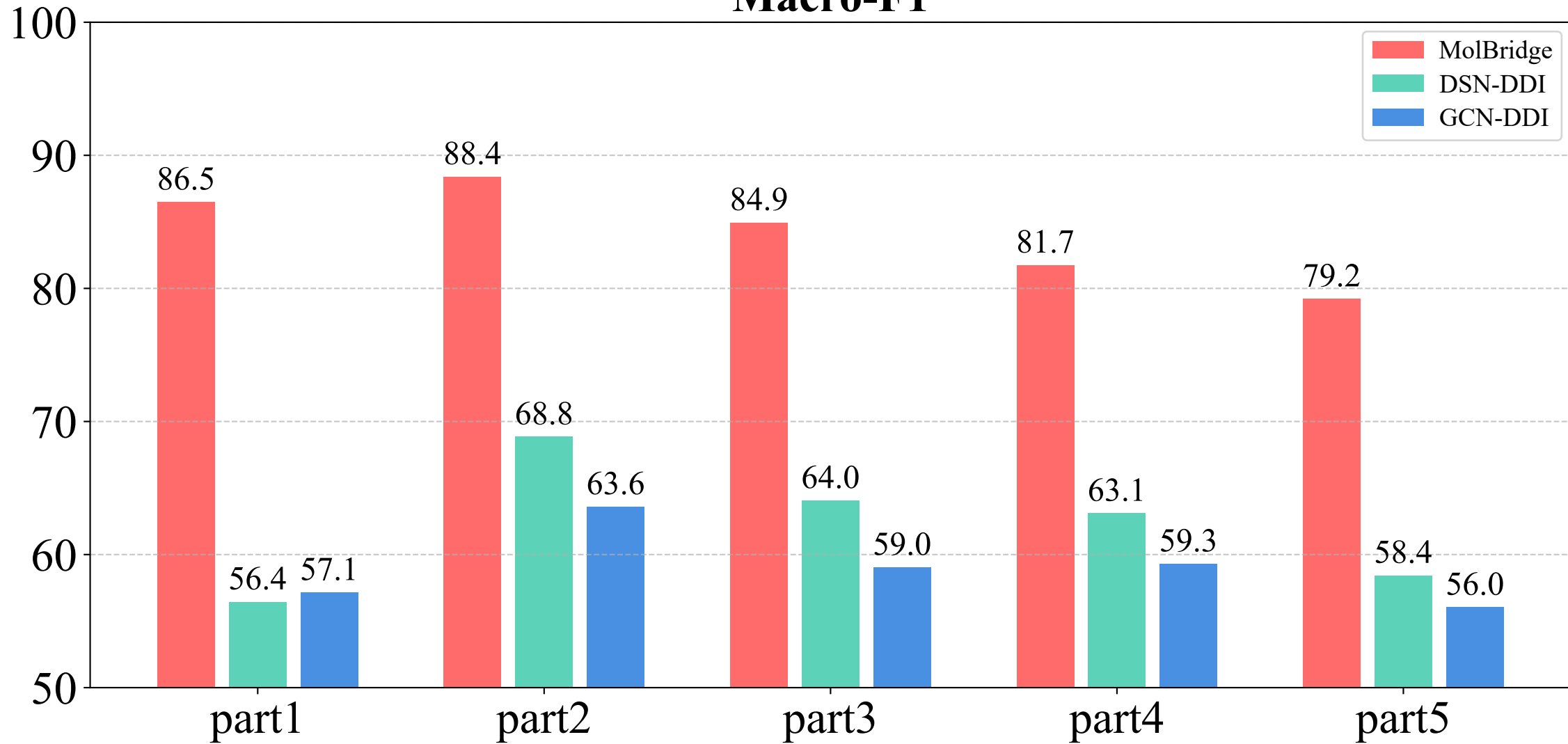
Macro-F1
