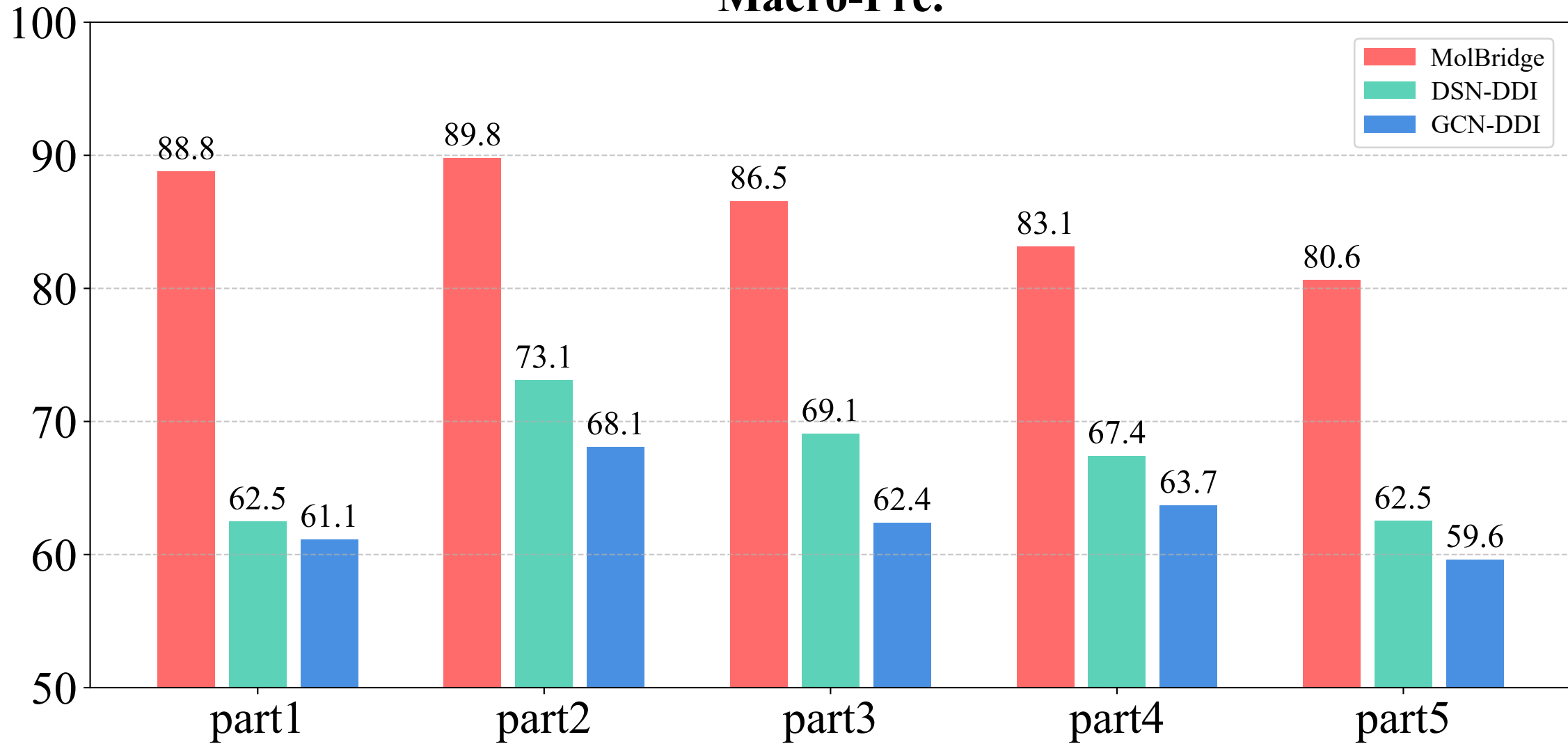
Macro-Pre.
