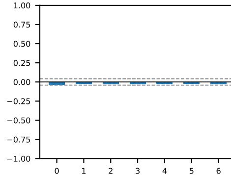
DGS2_diff(t-k) -&gt; VIXCLS(t)
