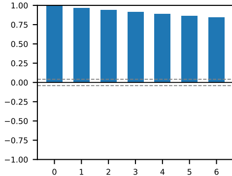
VIXCLS(t-k) -&gt; VIXCLS(t)
