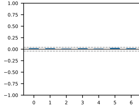
USEPUINDXD_diff(t-k) -&gt; VIXCLS(t)
