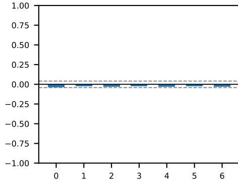
DEXUSEU_logreturn(t-k) -&gt; VIXCLS(t)
