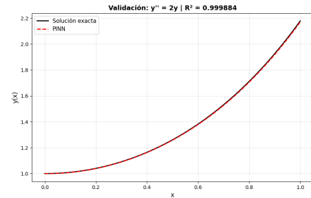
Figura 2. Gráfica comparativa de la solución de y'' = 2y mediante la PINN y su solución exacta
