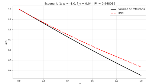
Figura 3. Aproximación de \delta(z) mediante PINN's para w = -1 y f_\nu = 0,04
