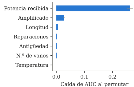
Fig. 3. Importancia de las variables por permutación (Random Forest, escenario B). Barras de error: desviación típica en 10 permutaciones.
