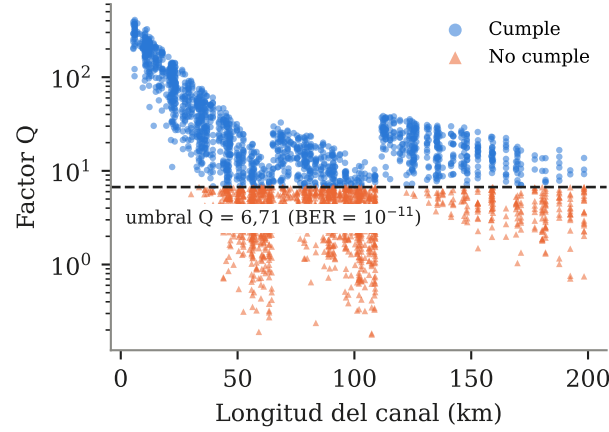
Fig. 1. Factor Q de cada canal según su longitud (muestra aleatoria de 1500 canales por clase); la línea discontinua es el umbral \text{BER} = 10^{-11} .
