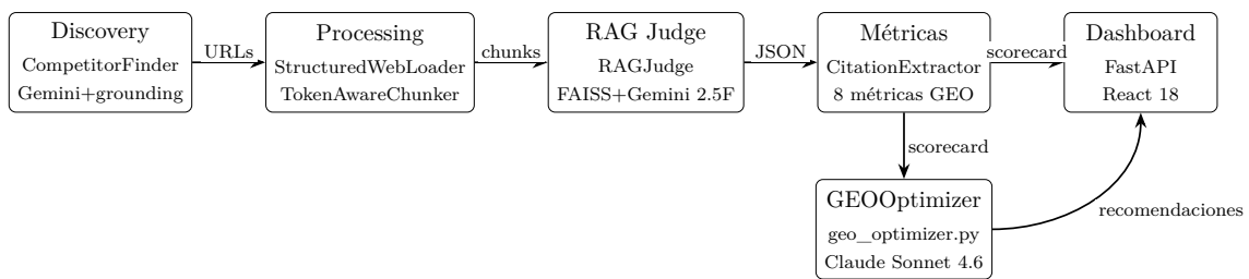
Figura 3.1: Diagrama de componentes del pipeline GEO-Audit.
