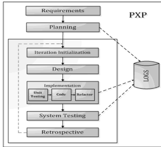
Figura 2.1: Diagrama de las fases de metodología Personal Extreme Programming (PXP) [17]
