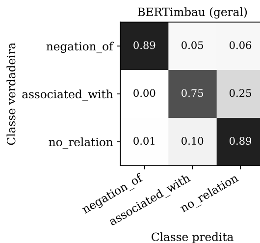
Figura 3. Matriz de confusão do BERTimbau (geral), normalizada por linha.
