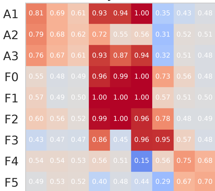
Layer 25
