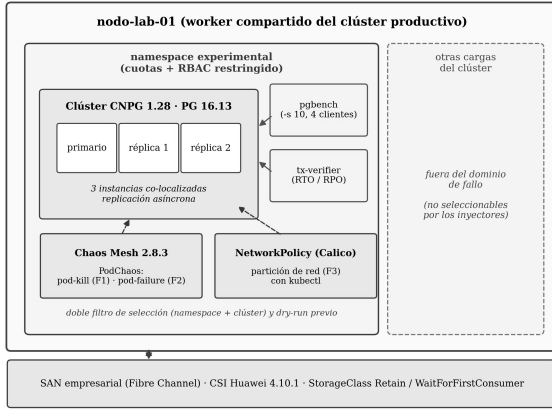
Fig. 1. Banco de pruebas: clúster experimental colocalizado en nodo-lab-01 , con clientes de carga ( pgbench ) y verificación ( tx-verifier ), e inyectores de fallo con doble filtro de selección; las cargas productivas quedan fuera del dominio de fallo.
