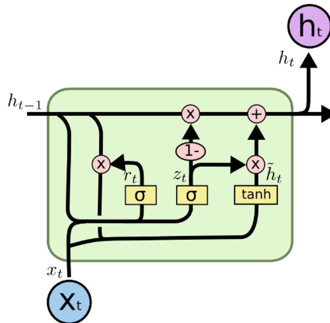
GRU
