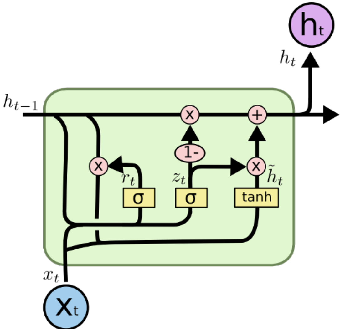
GRU
