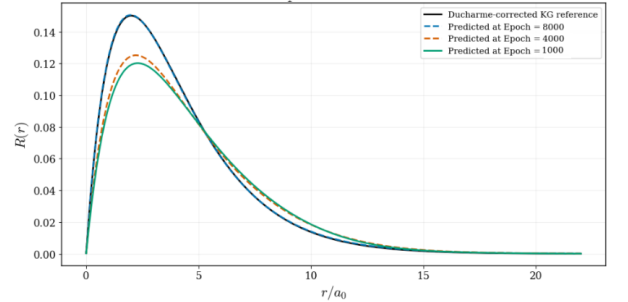
Figura 4: Solución radial R(r) para el estado 2p_{1/2} .
