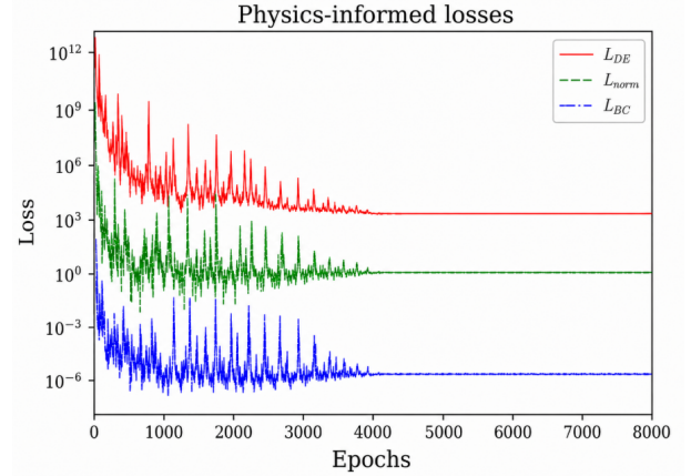
Figura 12: Evolución de las pérdidas físicas \mathcal{L}_{DE} , \mathcal{L}_{\text{norm}} y \mathcal{L}_{BC} durante el entrenamiento para el estado 3p_{3/2} .
