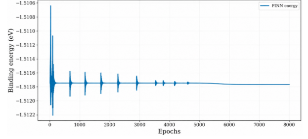
Figura 11: Evolución de la energía de ligadura aprendida por la PINN para el estado 3p_{3/2} .
