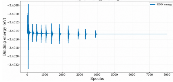
Figura 6: Evolución de la energía de ligadura aprendida por la PINN para el estado 2p_{1/2} .
