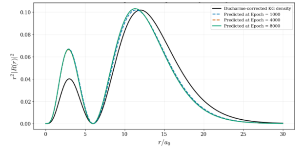
Figura 13: Densidad radial r^2|R(r)|^2 para el estado 3p_{3/2} , comparando la referencia KG–Ducharme con las predicciones de la PINN.
