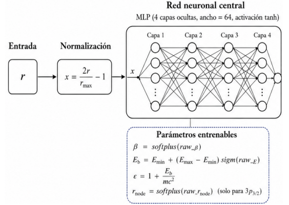
Figura 3: Arquitectura de la red neuronal informada por la física empleada para resolver el problema radial de autovalores asociado a la ecuación de Klein–Gordon corregida tipo Ducharme.
