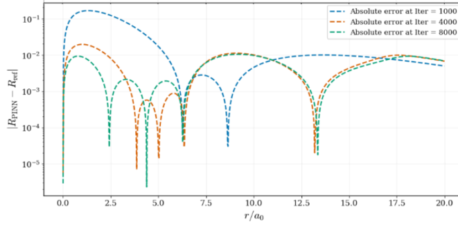
Figura 10: Error absoluto |R_{\text{PINN}} - R_{\text{ref}}| para el estado 3p_{3/2} en diferentes épocas de entrenamiento.
