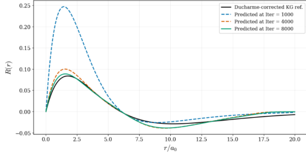
Figura 9: Solución radial R(r) para el estado 3p_{3/2} . Se comparan las predicciones de la PINN en diferentes épocas con la referencia KG–Ducharme.
