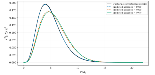
Figura 8: Densidad radial r^2|R(r)|^2 para el estado 2p_{1/2} , comparando la referencia KG–Ducharme con las predicciones de la PINN.
