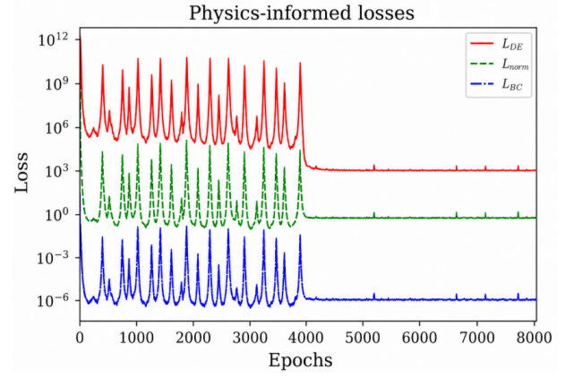
Figura 7: Evolución de las pérdidas físicas \mathcal{L}_{DE} , \mathcal{L}_{\text{norm}} y \mathcal{L}_{BC} durante el entrenamiento para el estado 2p_{1/2} para 8000 épocas.
