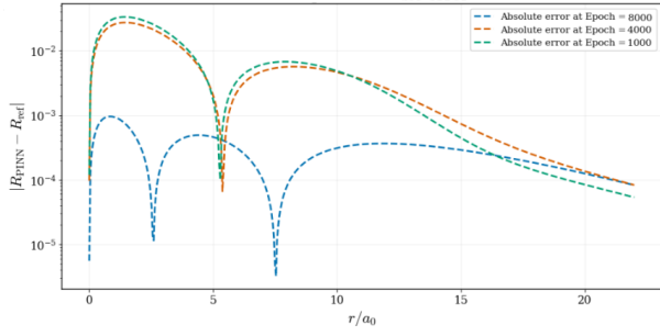
Figura 5: Error absoluto |R_{\text{PINN}} - R_{\text{ref}}| para el estado 2p_{1/2} en diferentes épocas de entrenamiento.
