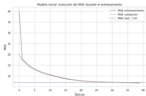
Figura 5. MAE durante el entrenamiento y test. [3]
