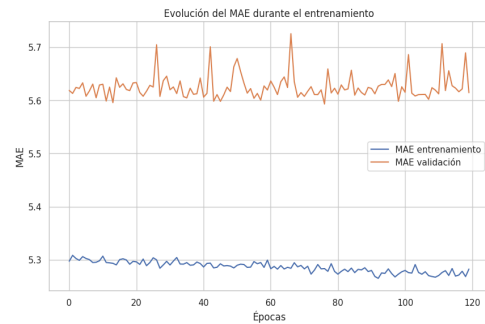
Figura 4. MAE durante el entrenamiento. [3]
