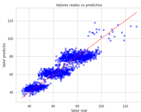
Figura 3 . Valores reales vs valores predichos [4]
