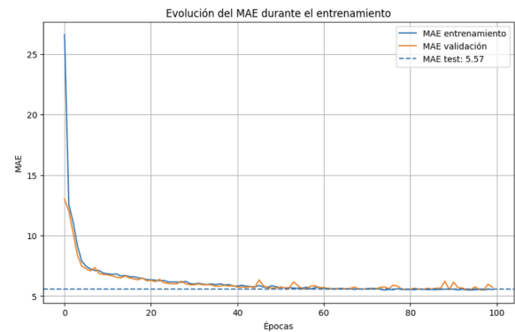
Figura 7. Evolución del MAE
