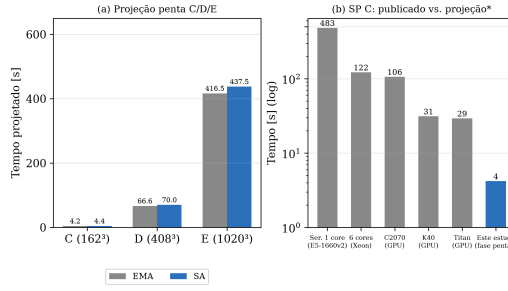
Figura 7. (a) Projeção da fase pentadiagonal para as classes C/D/E; (b) estado da arte publicado do SP C completo vs. projeção da fase pentadiagonal (asterisco: comparação por fase, não por benchmark).
