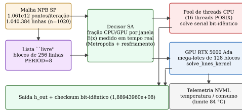
Figura 1. Arquitetura do solver híbrido: dispatcher com decisor SA, pool de threads CPU (EPYC 9124), mega-lotes de kernels GPU e telemetria NVML.
