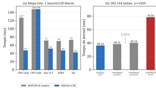
Figura 5. (a) Mega-lote vs. BATCH=8 por modo; (b) kernel de produção vs. cuPentBatch em 262.144 linhas (n=1020).
