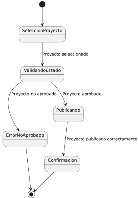
Diagrama de Estados - Publicación de Proyectos Aprobados
