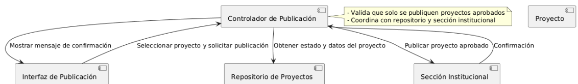
Diagrama de Componentes - Publicación de Proyectos Aprobados
