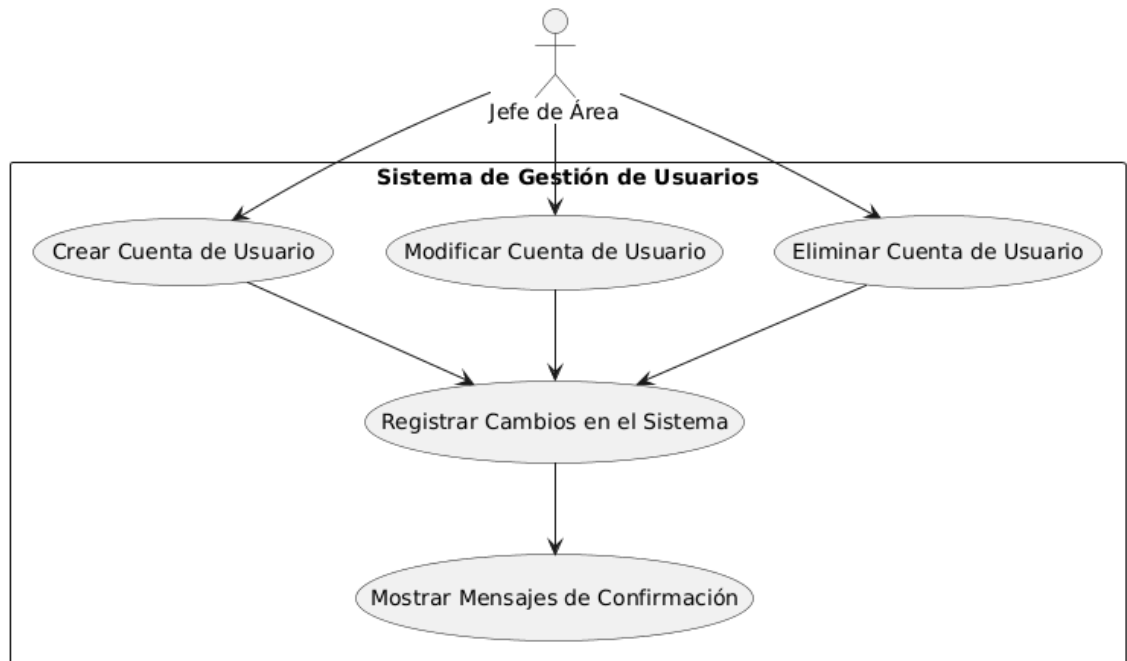
Diagrama de Casos de Uso - Gestión de Cuentas de Usuario
