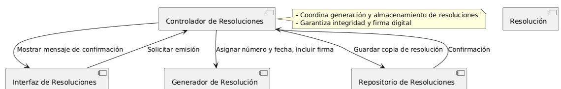
Diagrama de Componentes - Emisión de Resoluciones Digitales
