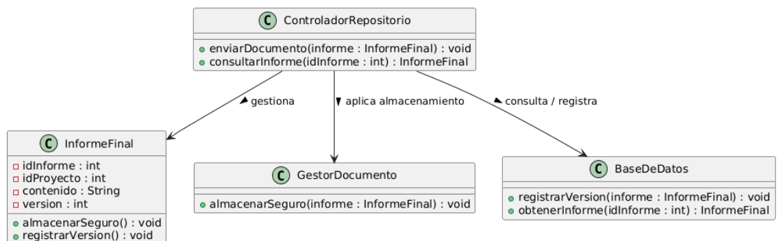
Diagrama de Clases - Almacenamiento de Informes Finales
