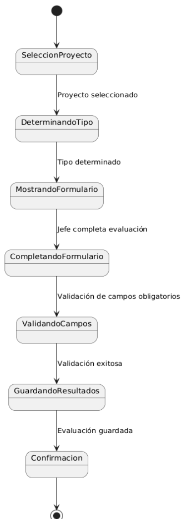
Diagrama de Estados - Formularios Según Tipo de Proyecto
