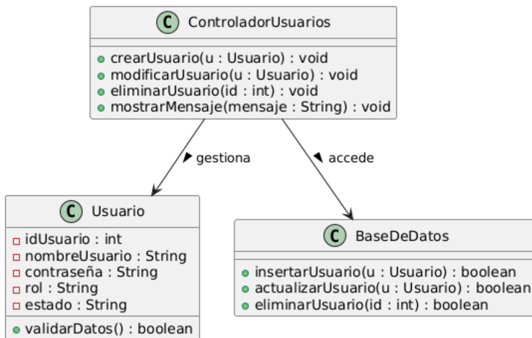
Diagrama de Clases - Gestión de Cuentas de Usuario
