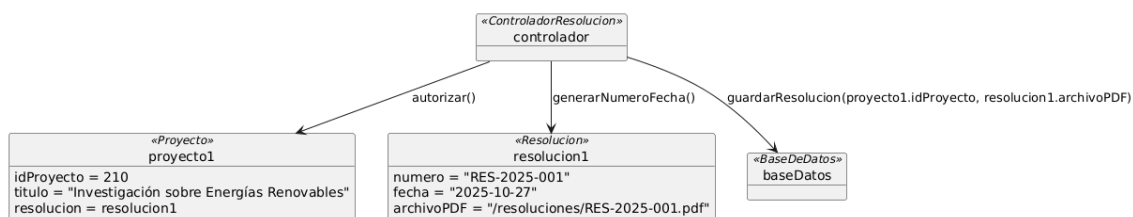
Diagrama de Objetos - Autorización de Proyectos
