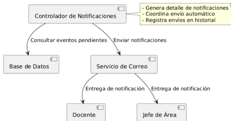
Diagrama de Componentes - Envío de Notificaciones Automáticas
