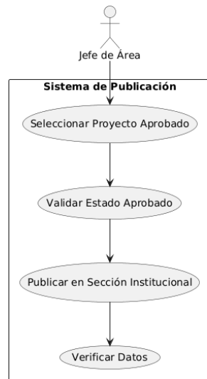
Diagrama de Casos de Uso - Publicación de Proyectos Aprobados
