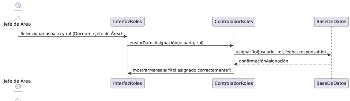
Diagrama de Secuencia - Asignación de Roles en el Sistema
