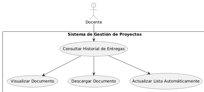
Diagrama de Casos de Uso - Consulta del Historial de Entregas
