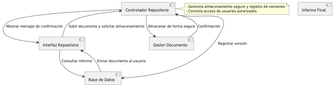
Diagrama de Componentes - Almacenamiento de Informes Finales
