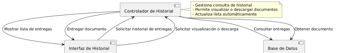
Diagrama de Componentes - Consulta del Historial de Entregas
