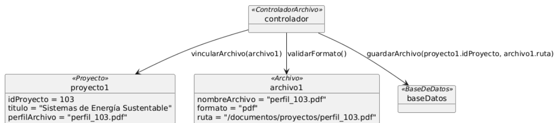
Diagrama de Objetos - Subida del Perfil del Proyecto
