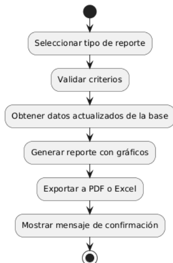
Diagrama de Actividad - Reportes Estadísticos
