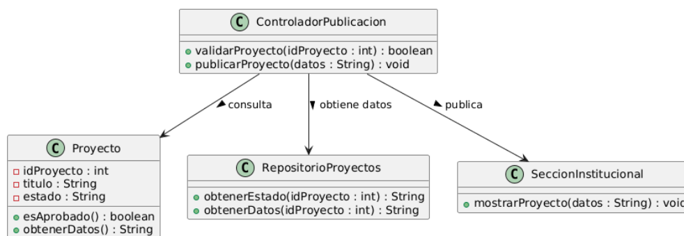
Diagrama de Clases - Publicación de Proyectos Aprobados
