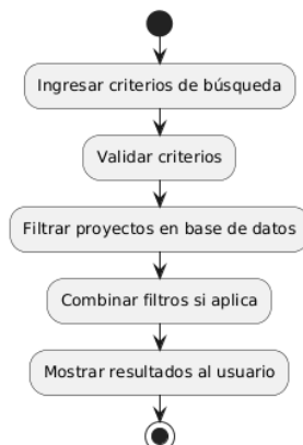
Diagrama de Actividad - Búsqueda y Filtrado de Proyectos
