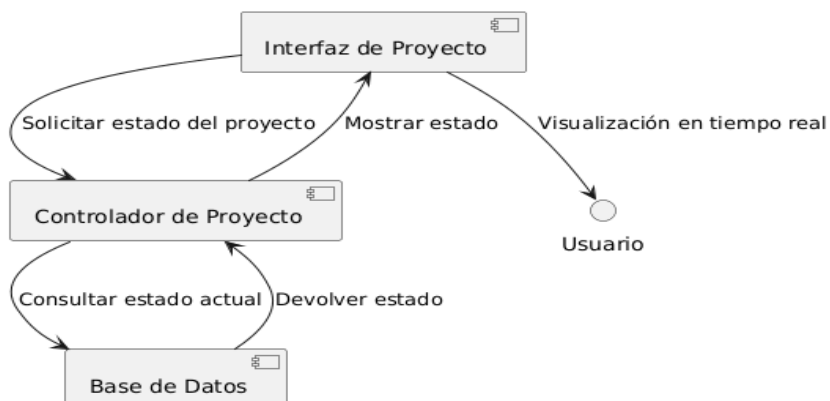
Diagrama de Componentes - Visualización del Estado del Proyecto
