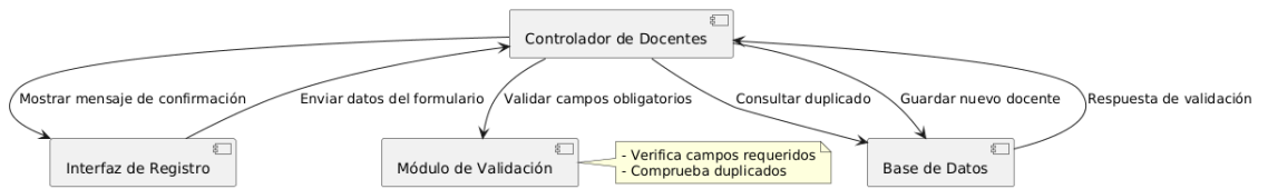
Diagrama de Componentes - Registro de Docentes Investigadores
