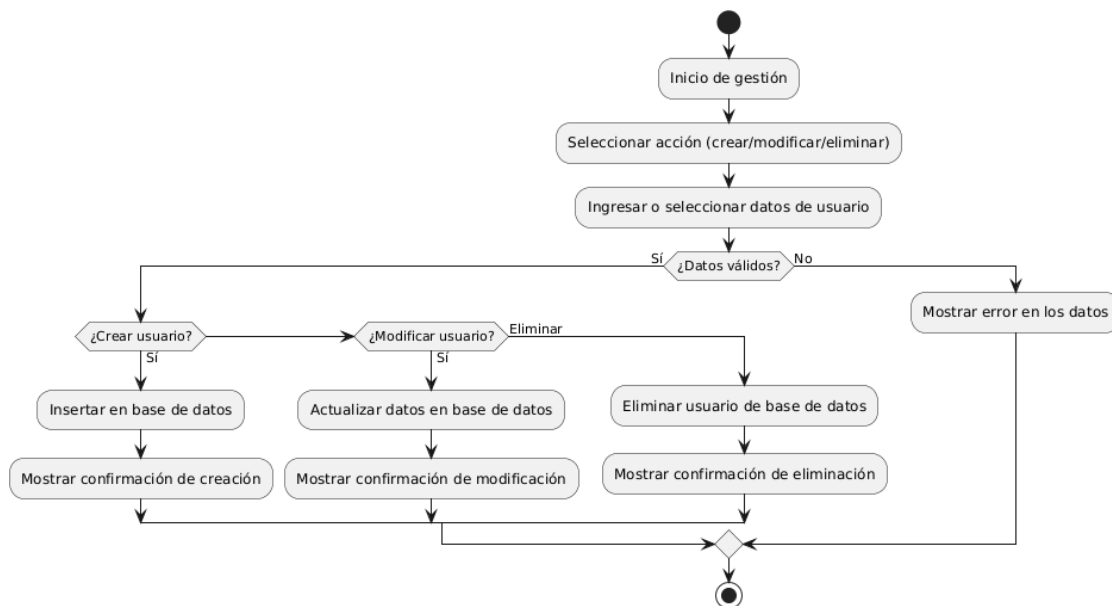
Diagrama de Actividad - Gestión de Cuentas de Usuario
