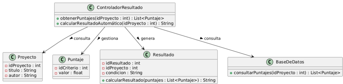
Diagrama de Clases - Cálculo Automático del Resultado
