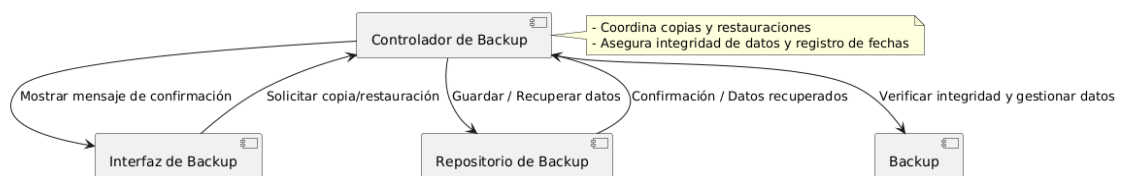
Diagrama de Componentes - Copias de Seguridad y Restauración
