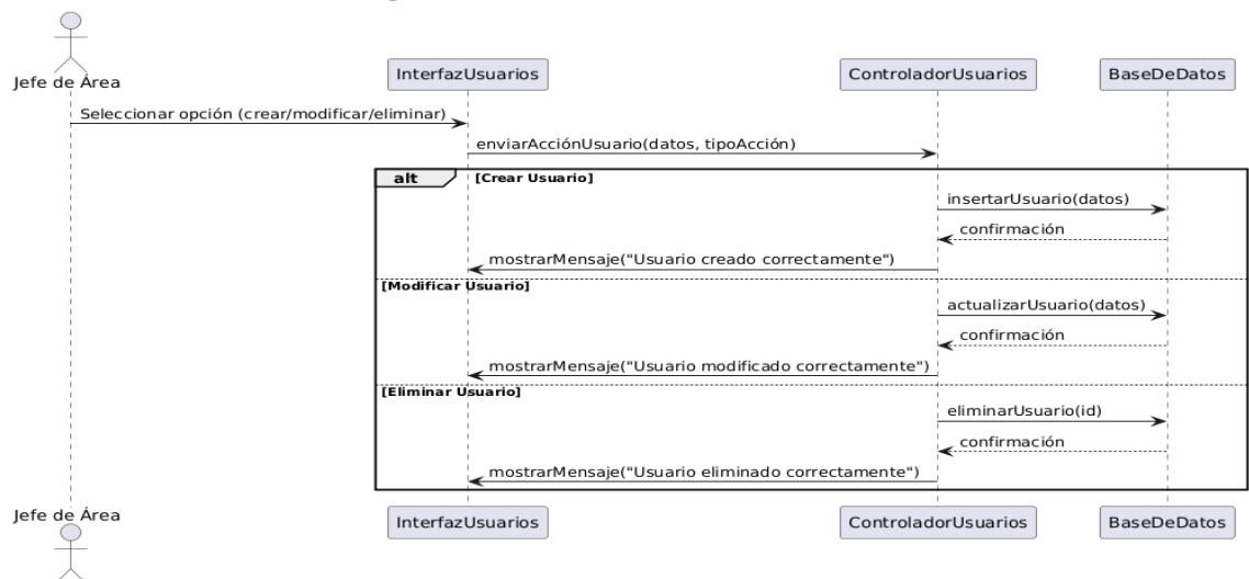
Diagrama de Secuencia - Gestión de Cuentas de Usuario
