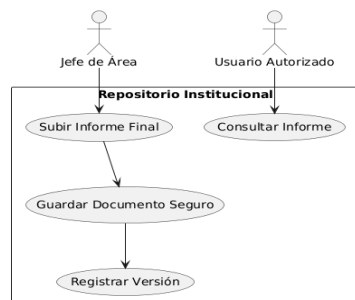
Diagrama de Casos de Uso - Almacenamiento de Informes Finales
