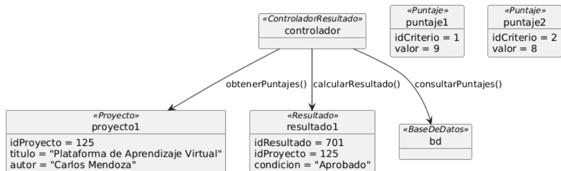
Diagrama de Objetos - Cálculo Automático del Resultado
