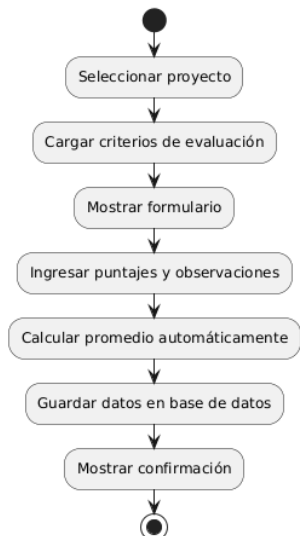
Diagrama de Actividad - Registro de Puntajes y Observaciones
