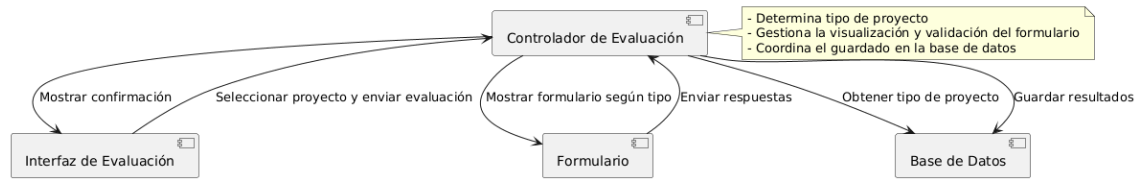
Diagrama de Componentes - Formularios Según Tipo de Proyecto
