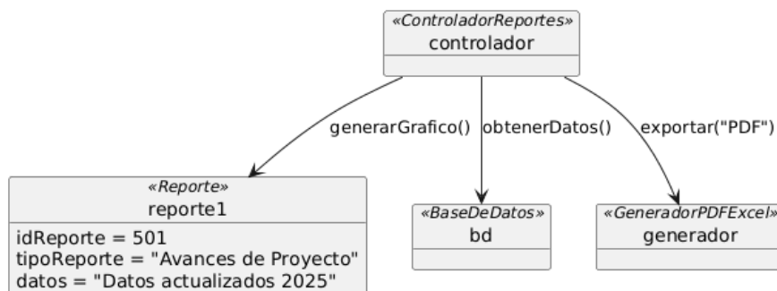
Diagrama de Objetos - Reportes Estadísticos
