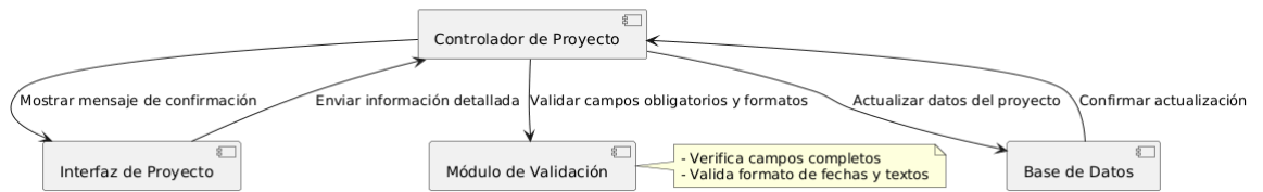
Diagrama de Componentes - Ingreso de Información Detallada del Proyecto
