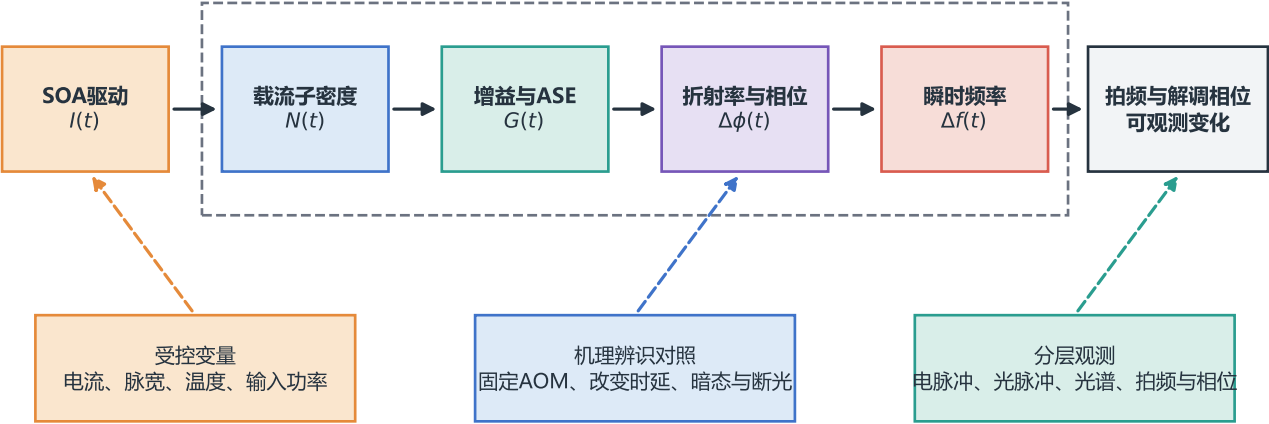
SOA载流子-折射率耦合的物理传递链与实验验证框架
