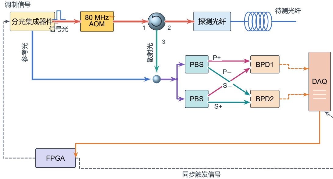
图 3-1 基于分光集成器件发射链路的偏振分集外差式 DAS 系统结构
