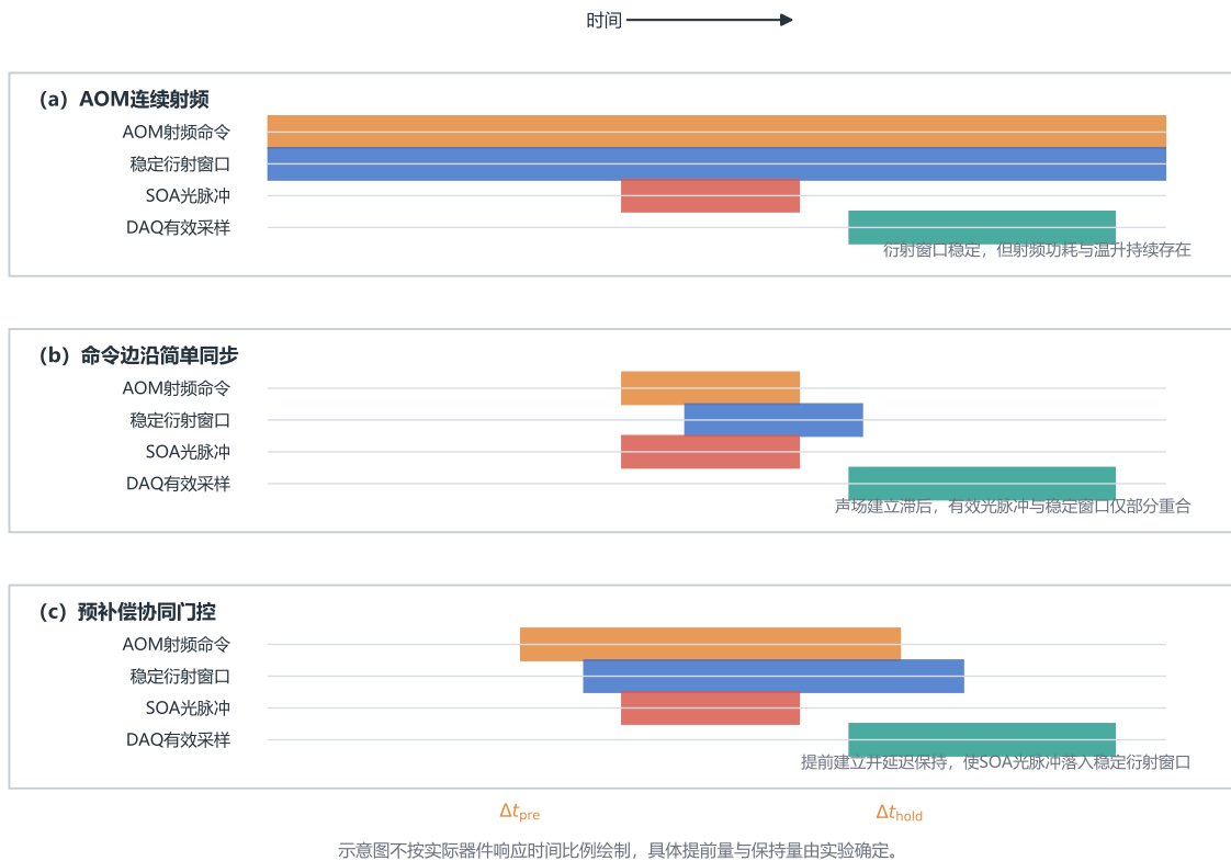
图 3-5 连续射频、命令边沿简单同步与预补偿协同门控的时序对比
