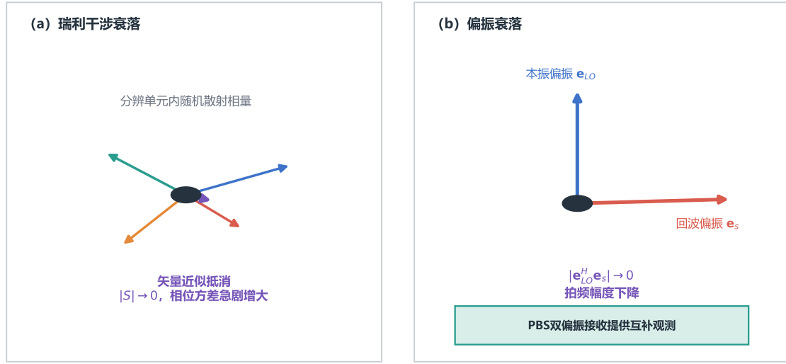
图 2-5 瑞利干涉衰落与外差相干接收中的偏振衰落机理
