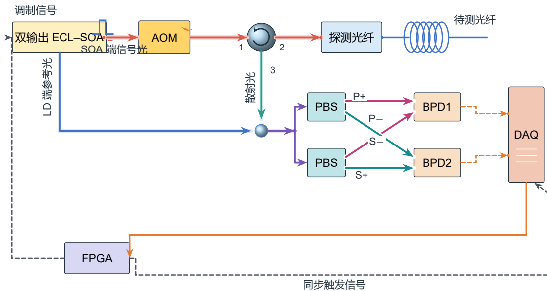
图 3-2 本文搭建的基于分光集成器件的分立式偏振分集 DAS 光路
