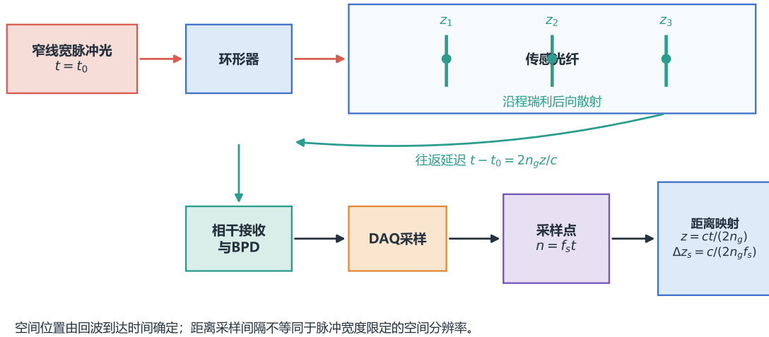
图 2-2 外差式 \phi -OTDR 瑞利后向散射与距离-时间映射示意图
