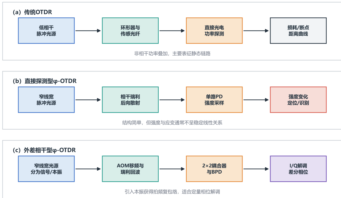
图 2-3 传统 OTDR、直接探测型与外差相干型 \varphi -OTDR 的信号链对比
