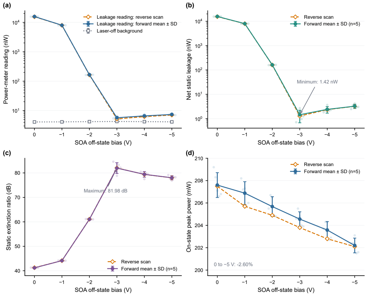
图 3-5 不同 SOA 关断反向偏压下的静态漏光与消光特性：(a) 漏光原始读数与暗态背景；(b) 扣除暗态背景后的净漏光功率；(c) 静态消光比；(d) 800 mA 导通脉冲峰值功率。浅色散点、实线误差棒与空心菱形虚线分别表示 5 轮正向扫描的单次结果、均值与标准差及反向扫描结果。
