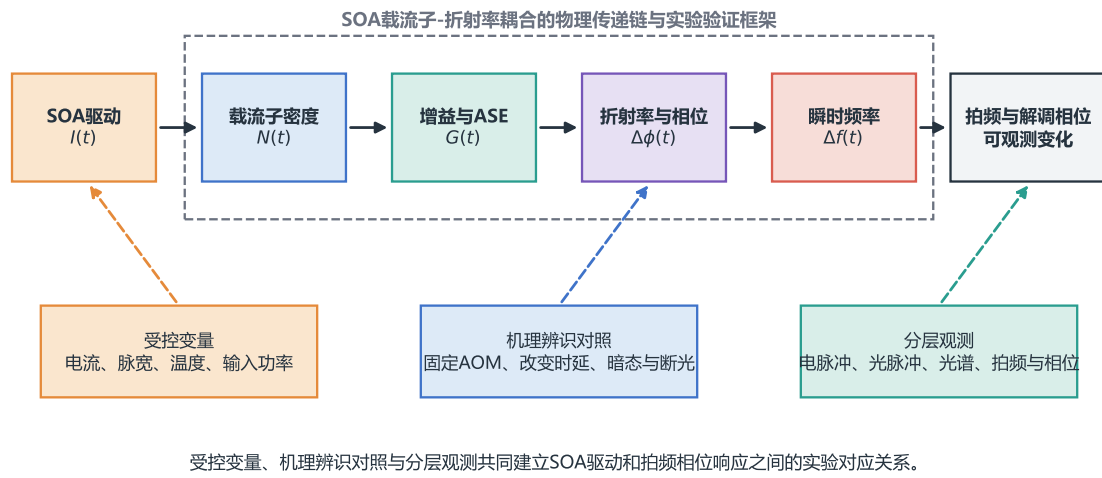
图 2-4 SOA 工作状态到外差拍频与解调相位的传递链路
