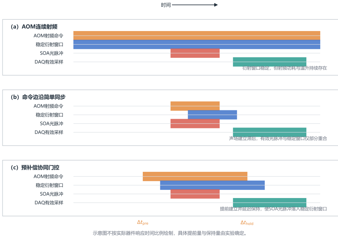
图 3-6 连续射频、命令边沿简单同步与预补偿协同门控的时序对比
