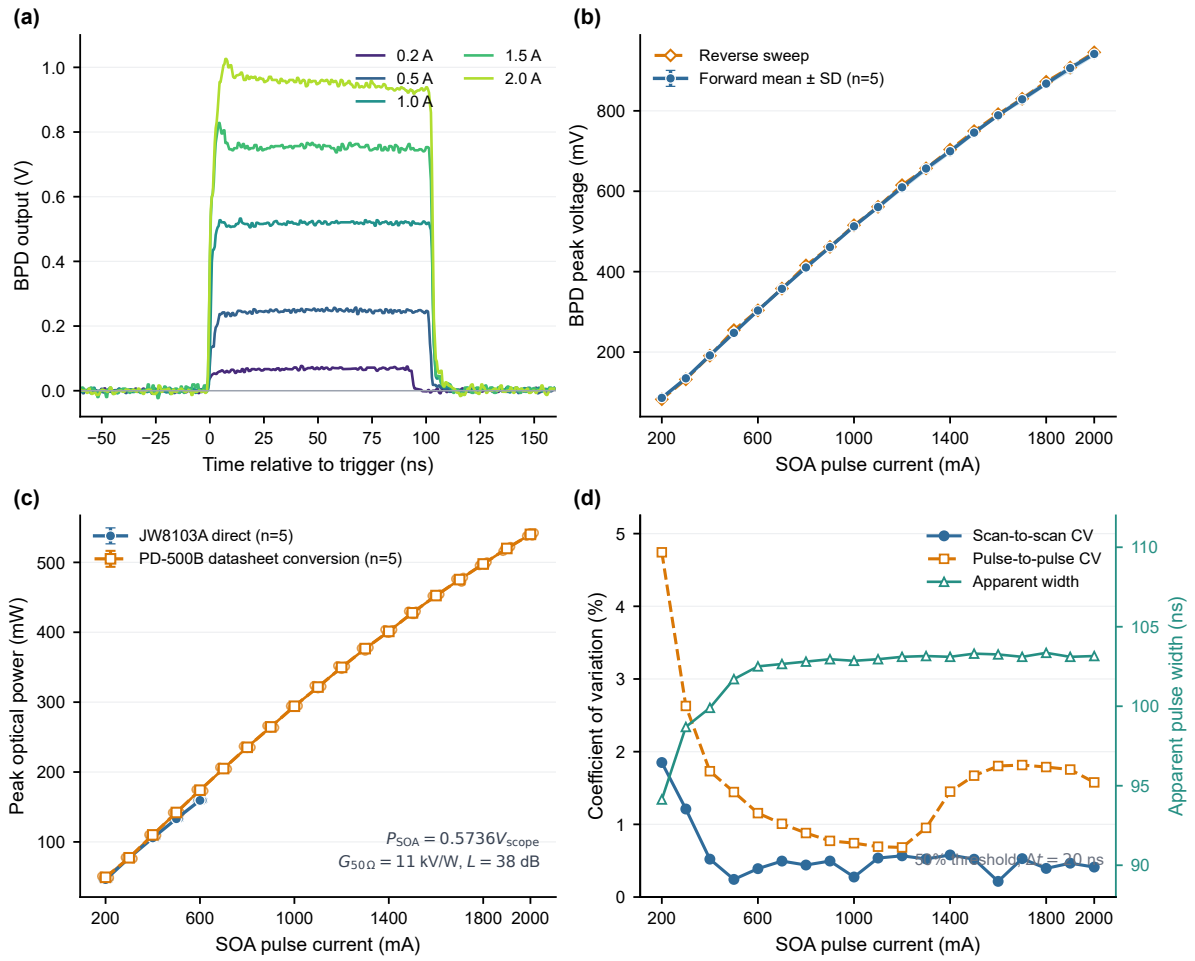
图 3-4 不同 SOA 脉冲电流下的输出脉冲与重复性表征：(a) 4 GSa/s 高分辨率单脉冲波形；(b) 5 轮正向扫描的 BPD 峰值电压及反向扫描结果；(c) 由 PD-500B 规格增益和 38 dB 总衰减计算的峰值光功率及功率计独立校核值；(d) 399 脉冲长记录所得跨轮与脉冲间变异系数及 50% 阈值表观脉宽。
