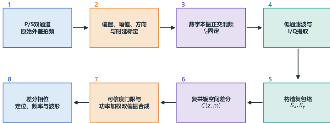
该流程统一了原始拍频信号至差分相位的数据处理步骤。
