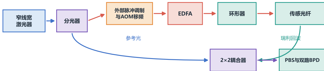
(a) 传统EDFA分立光路
