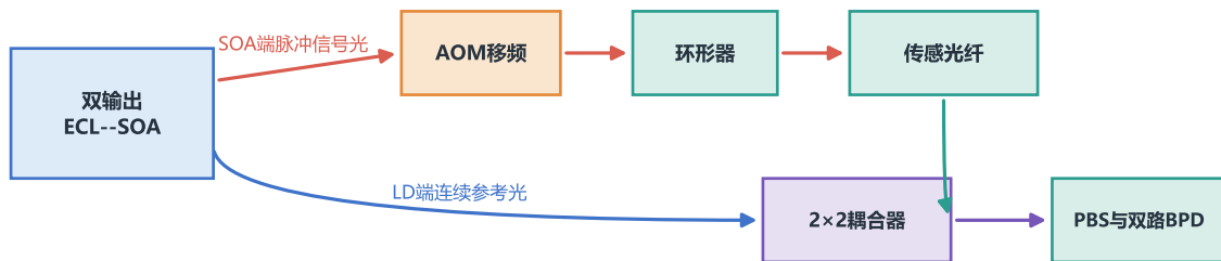
(b) 本文双输出ECL--SOA光路
