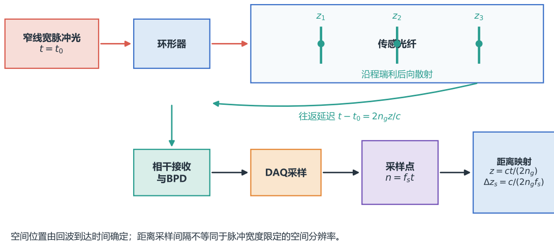
图 2-2 外差式 \varphi -OTDR 瑞利后向散射与距离-时间映射示意图
