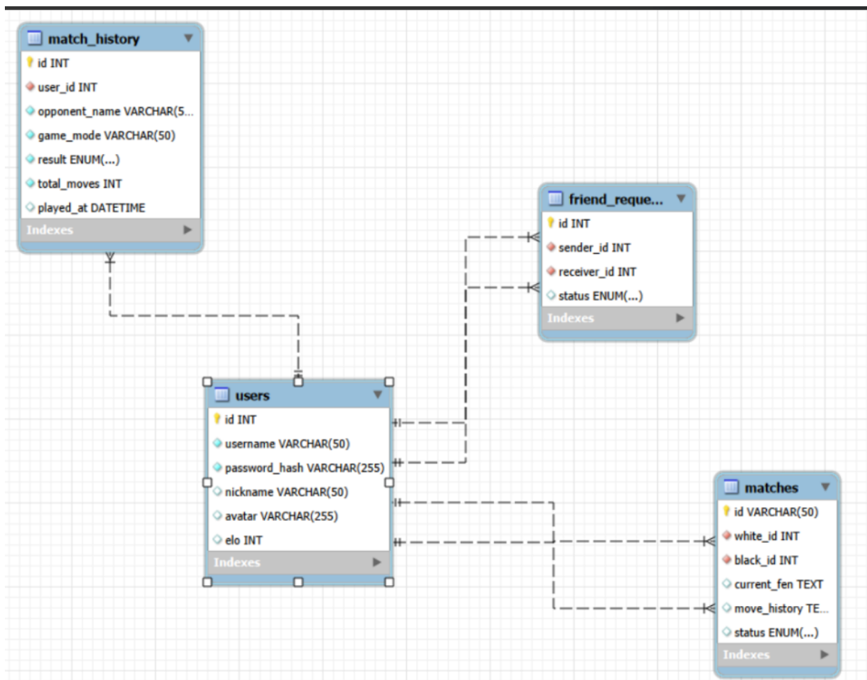
Hình 3.2: Sơ đồ Thực thể liên kết (ERD) mô tả mối quan hệ giữa các bảng
