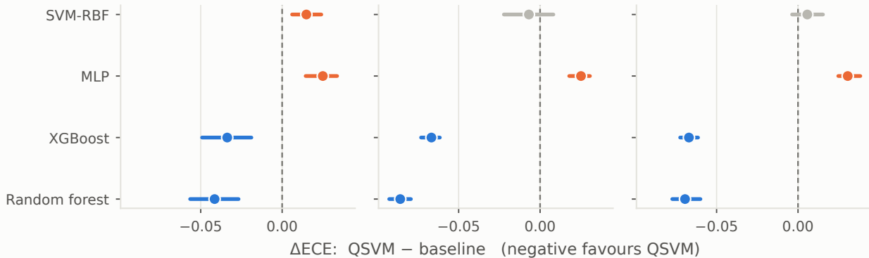
NSL-KDD 4 qubits
