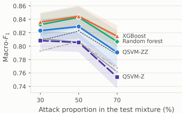
(a) Class-prior shift
