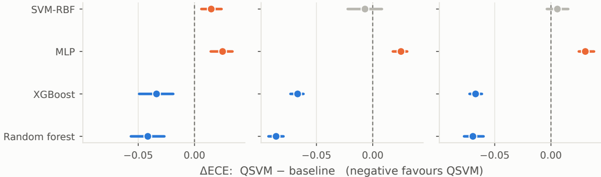
NSL-KDD 4 qubits
