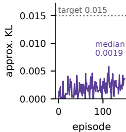
(d) PPO update size
