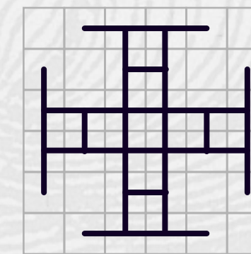
另一者
