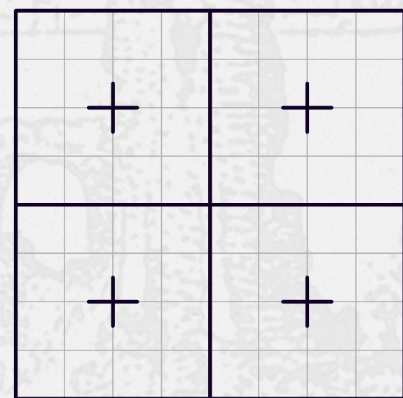
8阶
