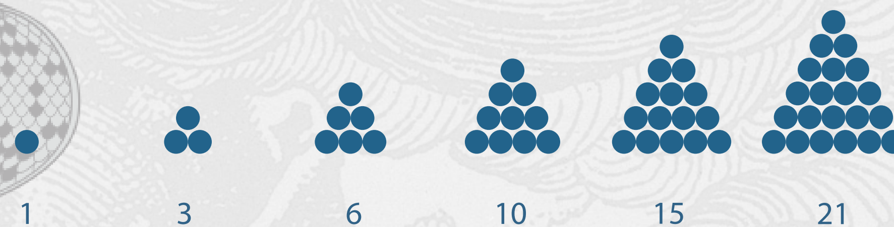
三角形数
