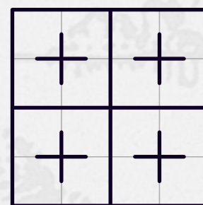
4阶
