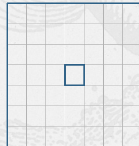
7阶
