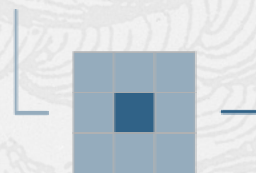
1 同构
