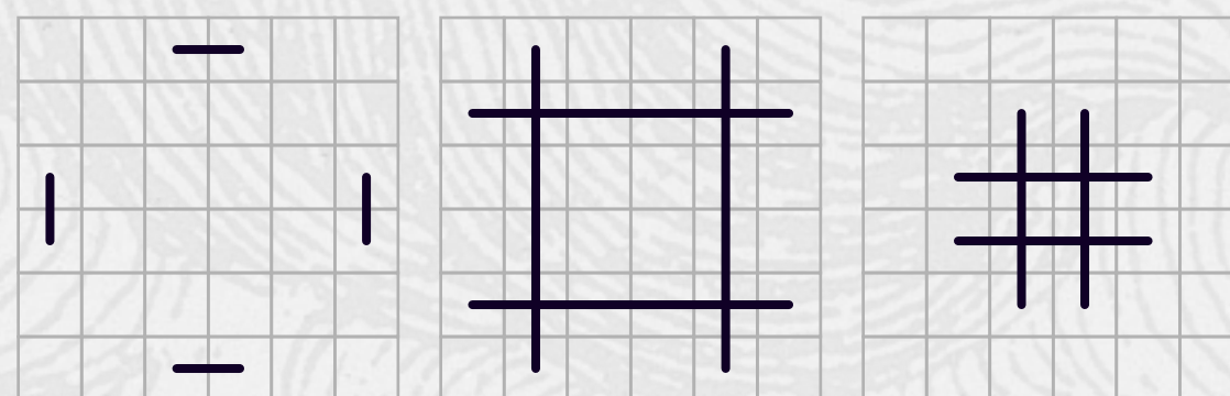
自我
