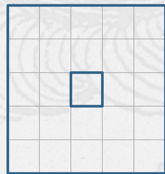
5阶
