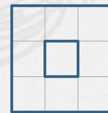
3阶
