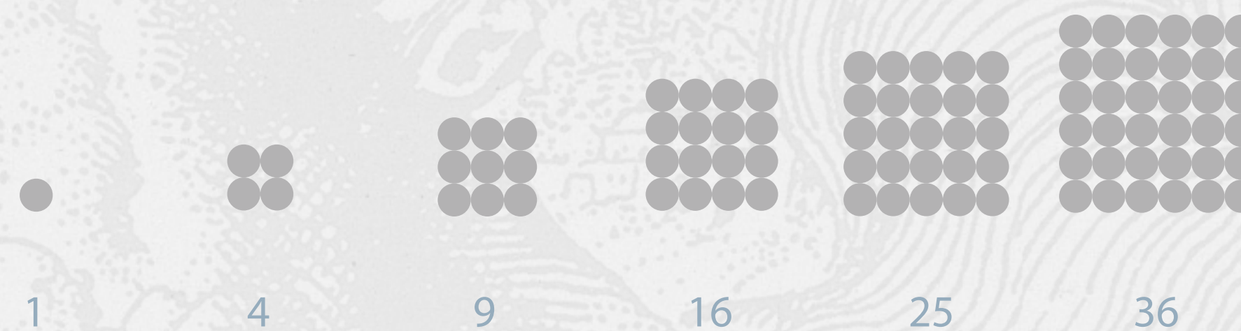
正方形数
