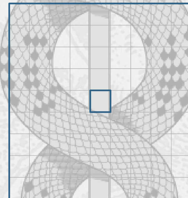
9阶
