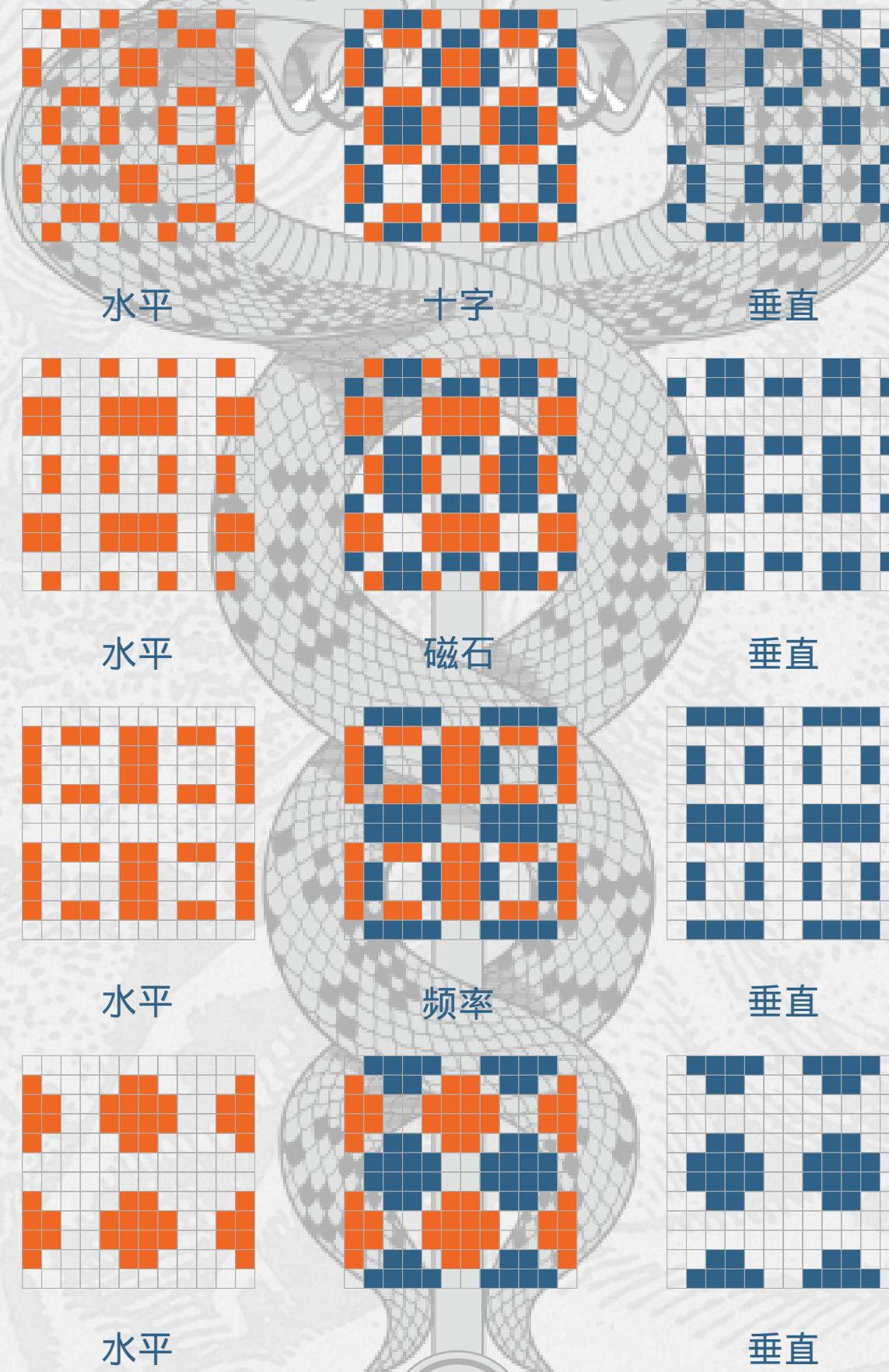
十二阶
