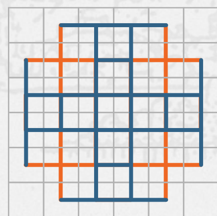
六阶
