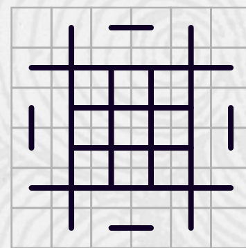
自我
