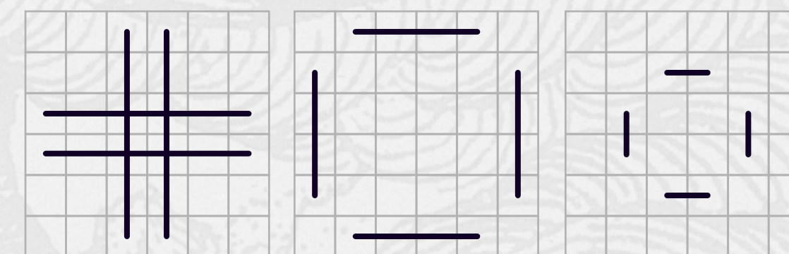
另一者
