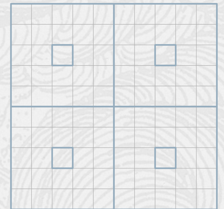
10阶
