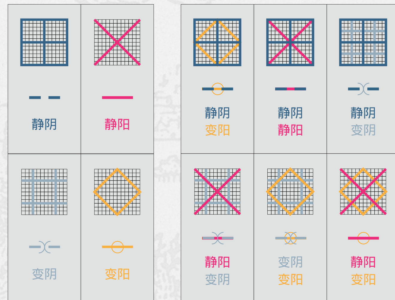
四种基础
