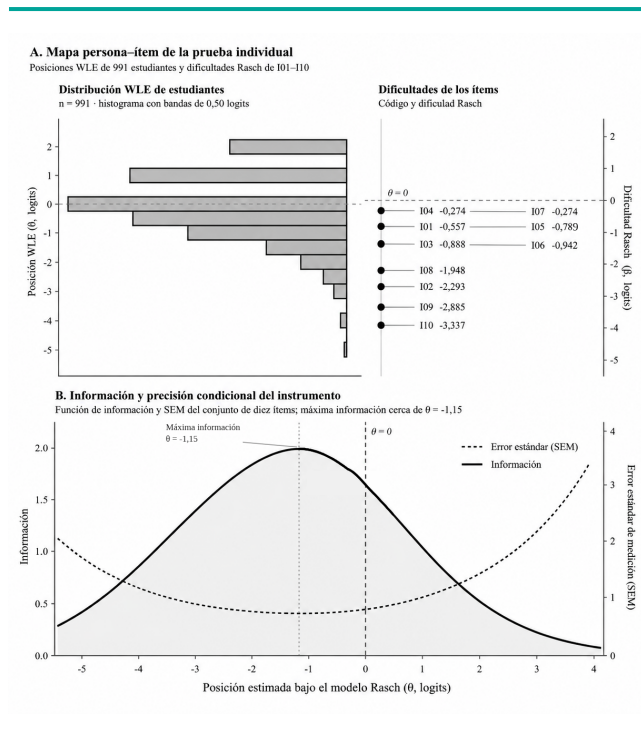
Figura 7. Focalización y precisión condicional de la prueba individual bajo el modelo de Rasch. El panel A presenta la distribución de las posiciones WLE de 991 estudiantes y las dificultades estimadas de los diez ítems sobre una escala común en logits. El panel B muestra la función de información del instrumento y el error estándar de medición (SEM) a lo largo del continuo. Las dificultades se concentran entre -3,337 y -0,274 logits y la máxima información se ubica aproximadamente en \theta = -1,15 , lo que muestra una mejor focalización hacia la zona baja-media que hacia posiciones altas del continuo.
