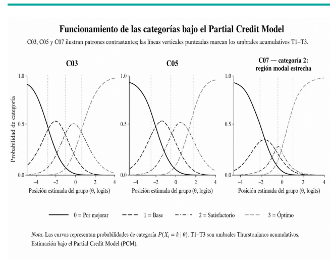
Figura 14. Funcionamiento de las categorías de puntuación bajo el Partial Credit Model. Se presentan las curvas de probabilidad de categoría para Co3, Co5 y Co7 como ejemplos de patrones contrastantes. Las cuatro categorías alcanzan una región modal propia en los ocho criterios dentro del rango de habilidad examinado. Co7 presenta la principal señal descriptiva para inspección adicional: la categoría 2 ( Satisfactorio ) posee una región modal comparativamente estrecha. Las líneas verticales punteadas indican los umbrales Thurstonianos acumulativos T1-T3.
